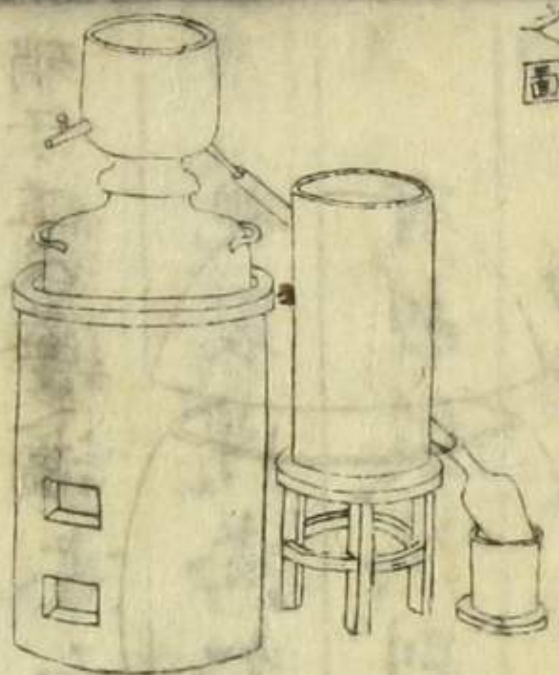
厲的兒篤安爐中行砂火法 之圖
