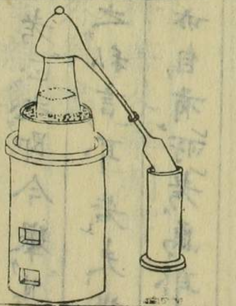
箇爾否行砂火法之圖
