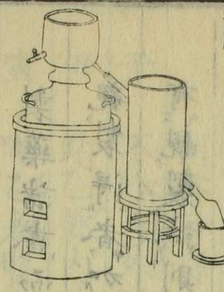
蒸露鐘安爐上接蛇管及壺之圖
