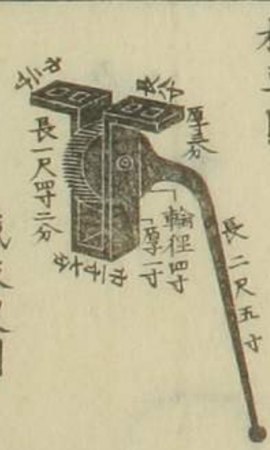
鐵板架圖
