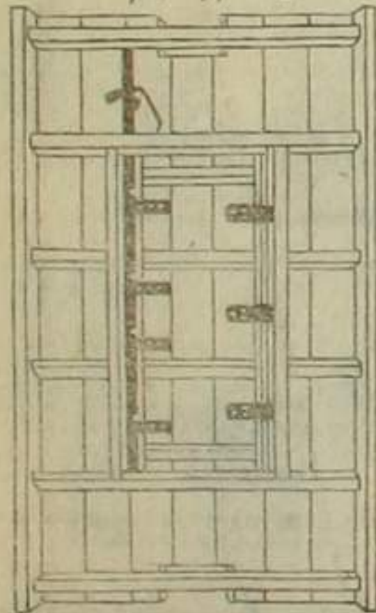
踏板裏面圖
