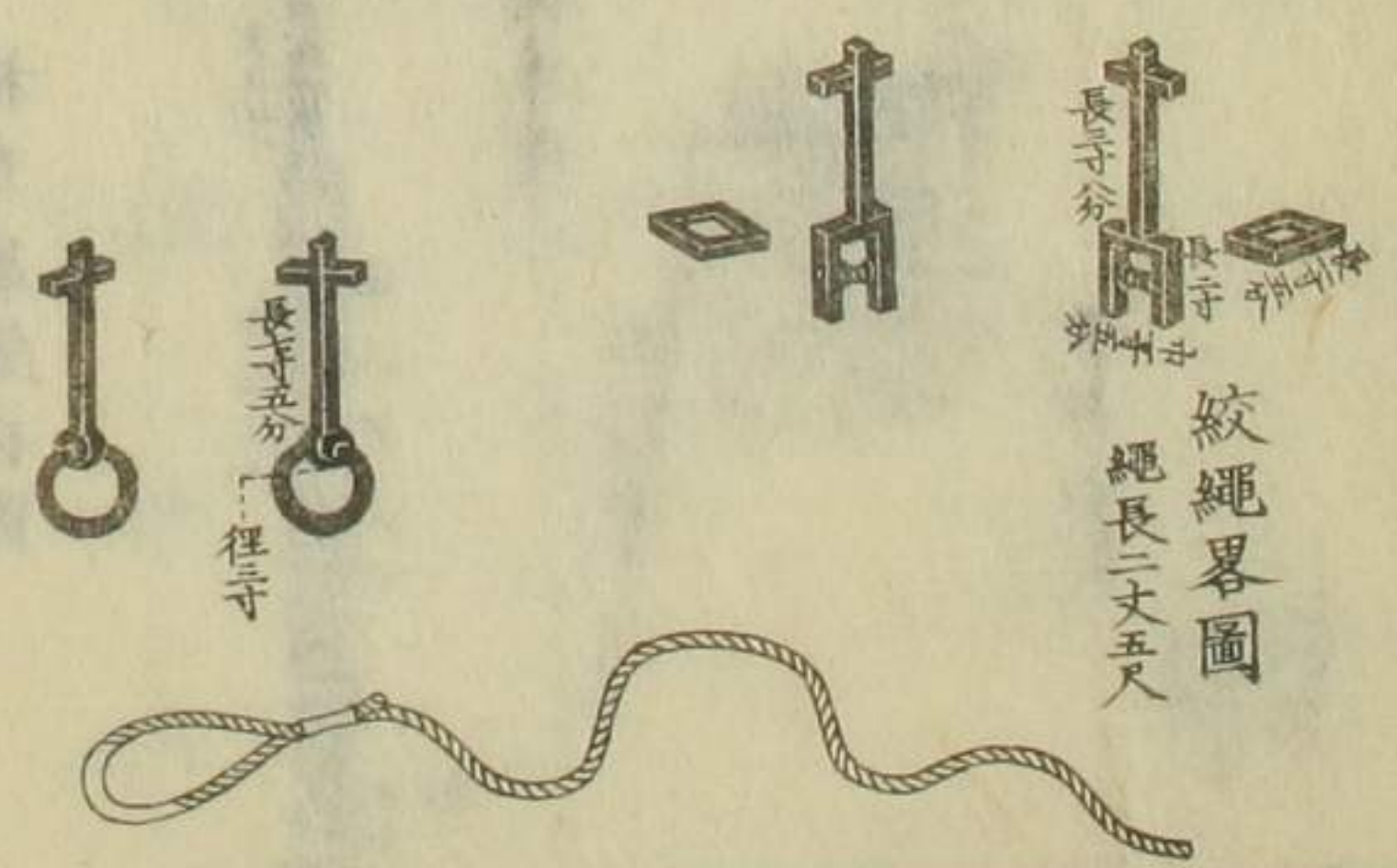
絞繩器圖
