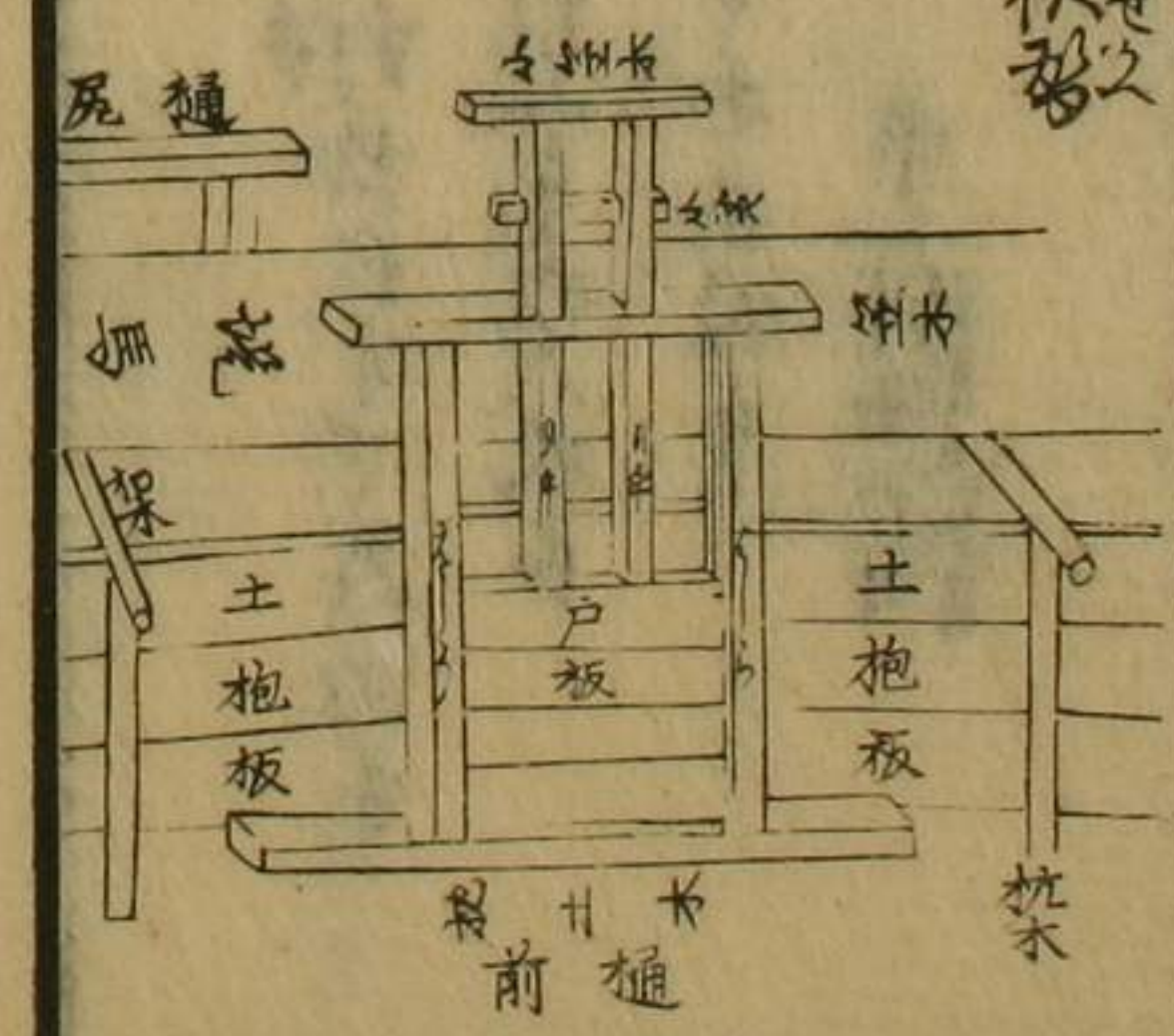
一戸前の以榎の圖
