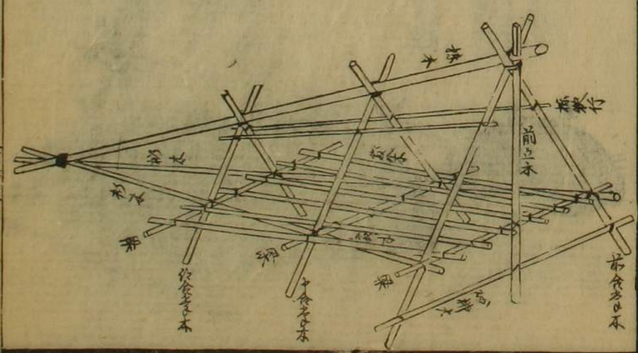
大工の 半架 の 圖
