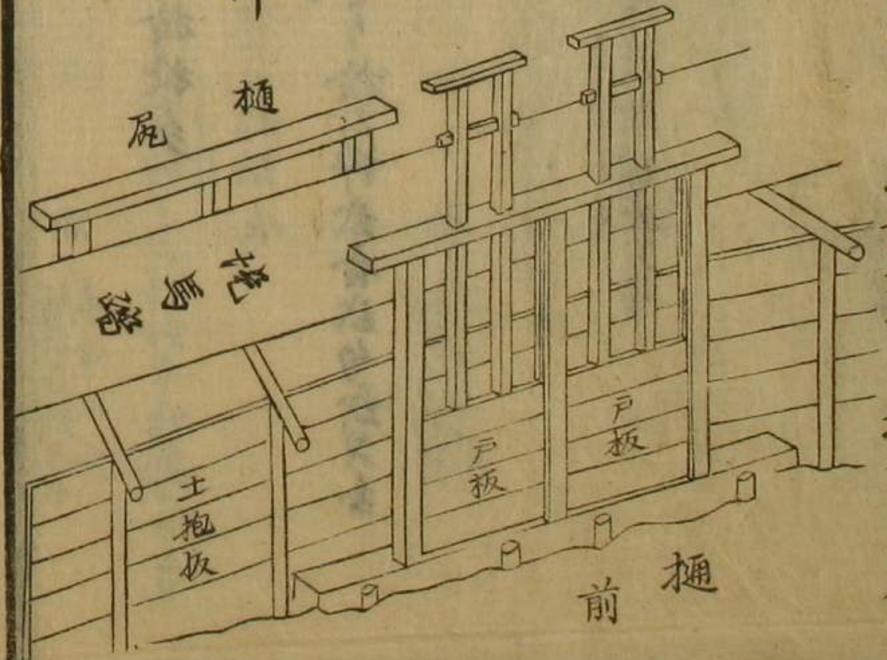
二戸 前坪 榎の圖
