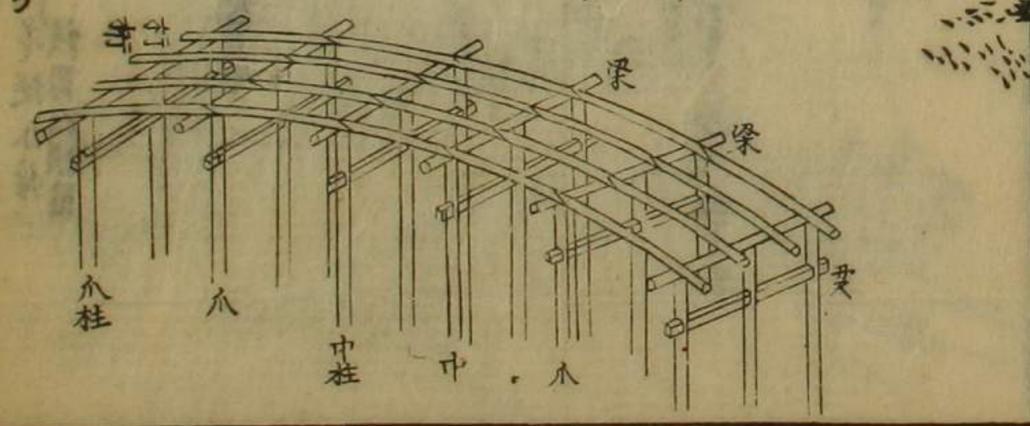
同橋柱の圖
