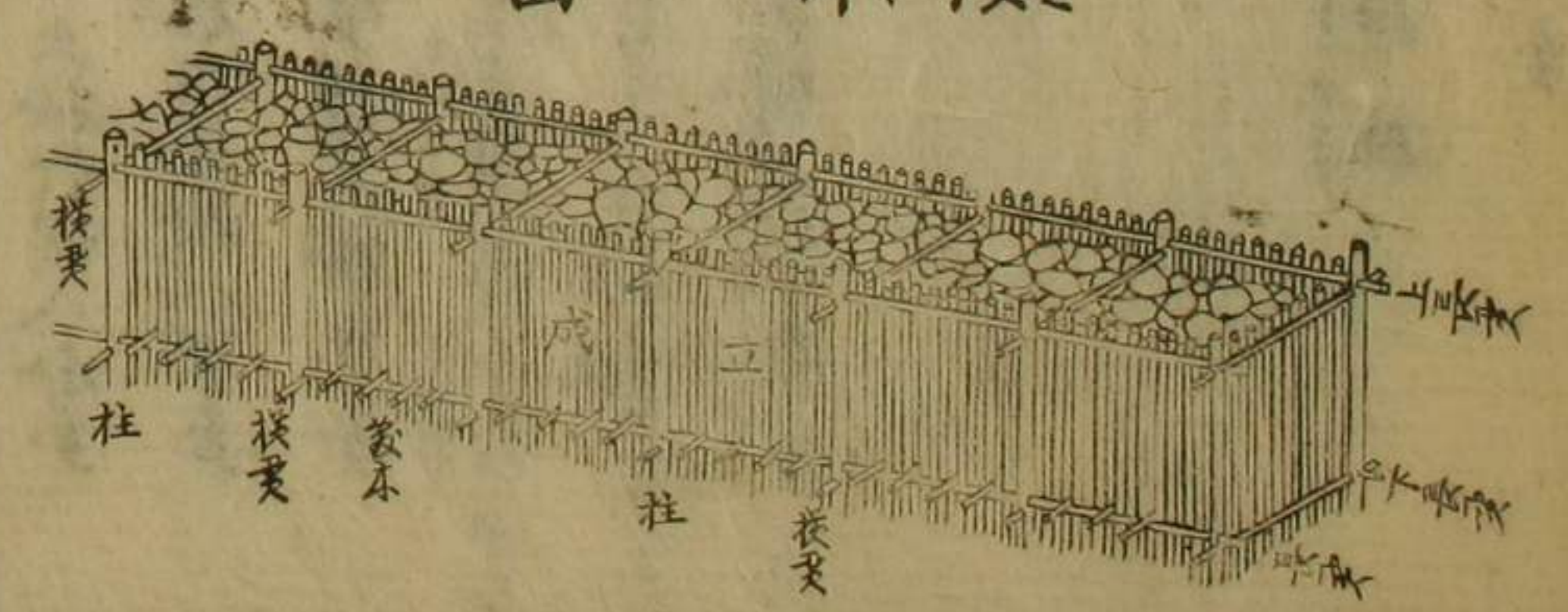
圖の棟續
