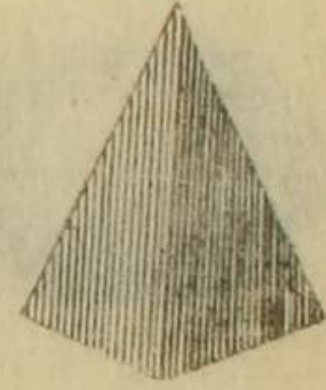
方錐體
