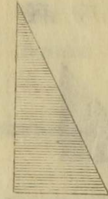
不等三角
