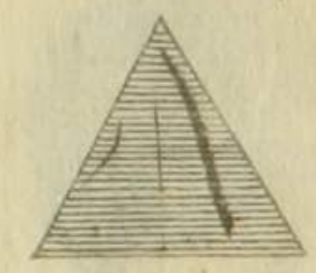
角三正
