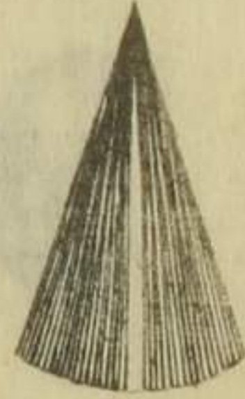
圓錐體
