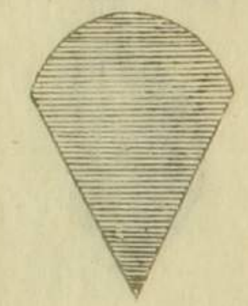
角三弧邊一
