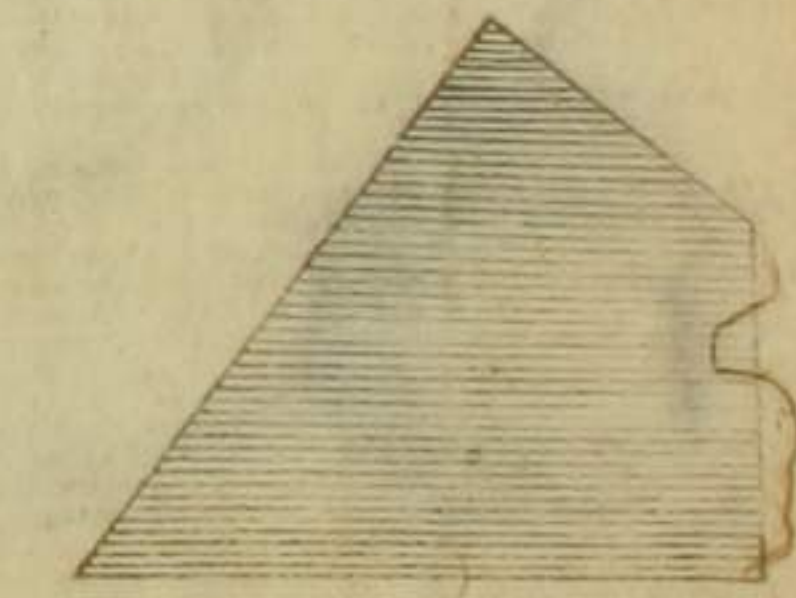
形方等不
