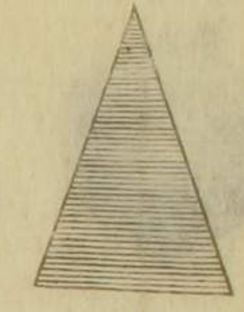
等脚三角
