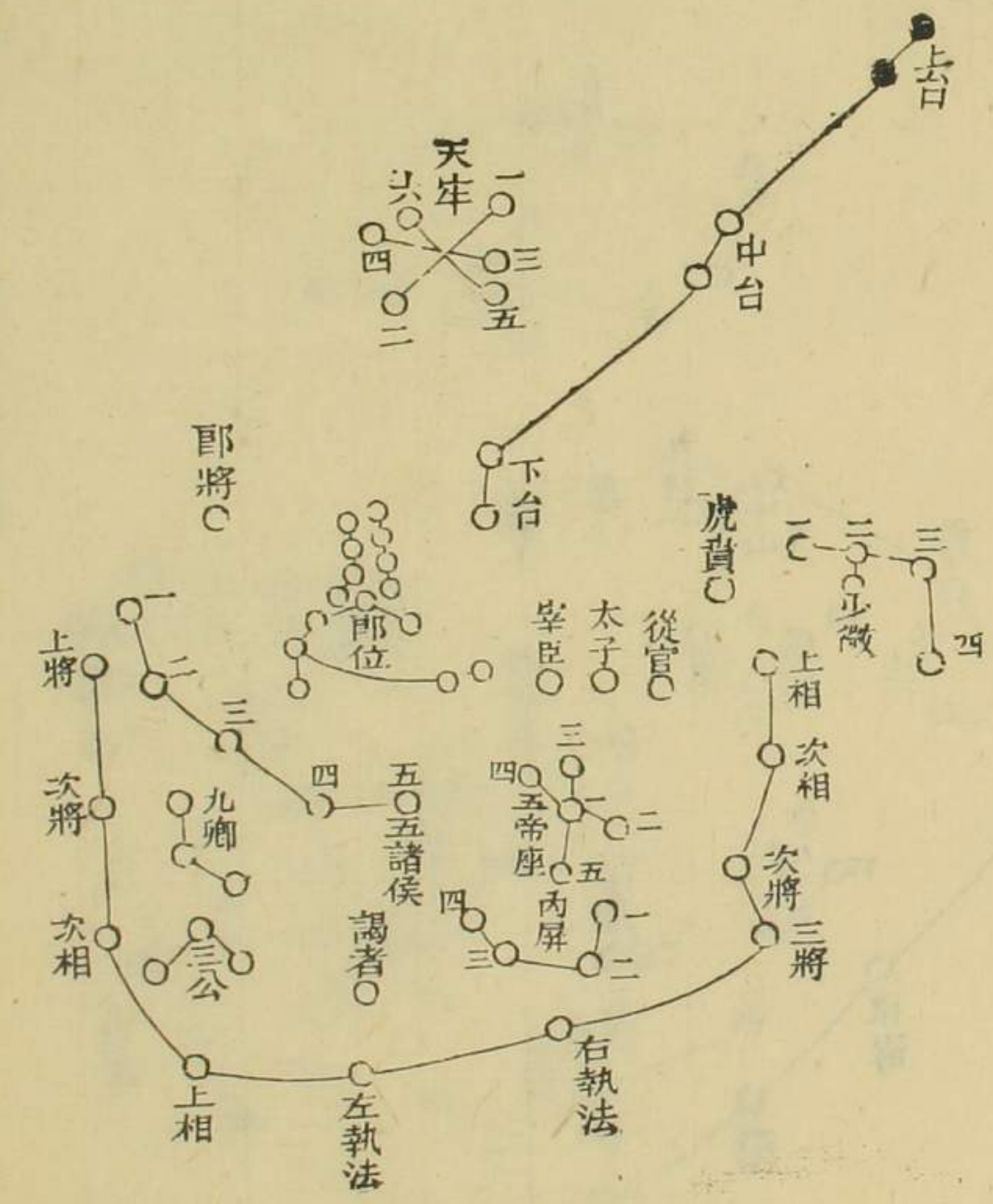
太微垣上台二星分楚圖
