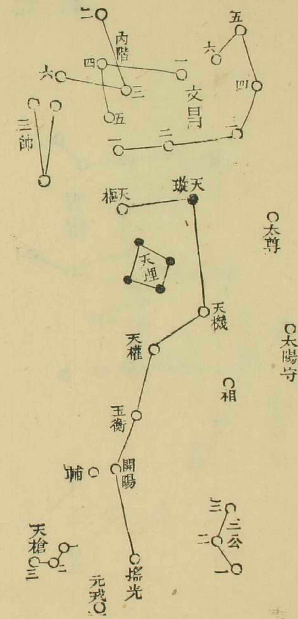
北斗第二星分楚圖
