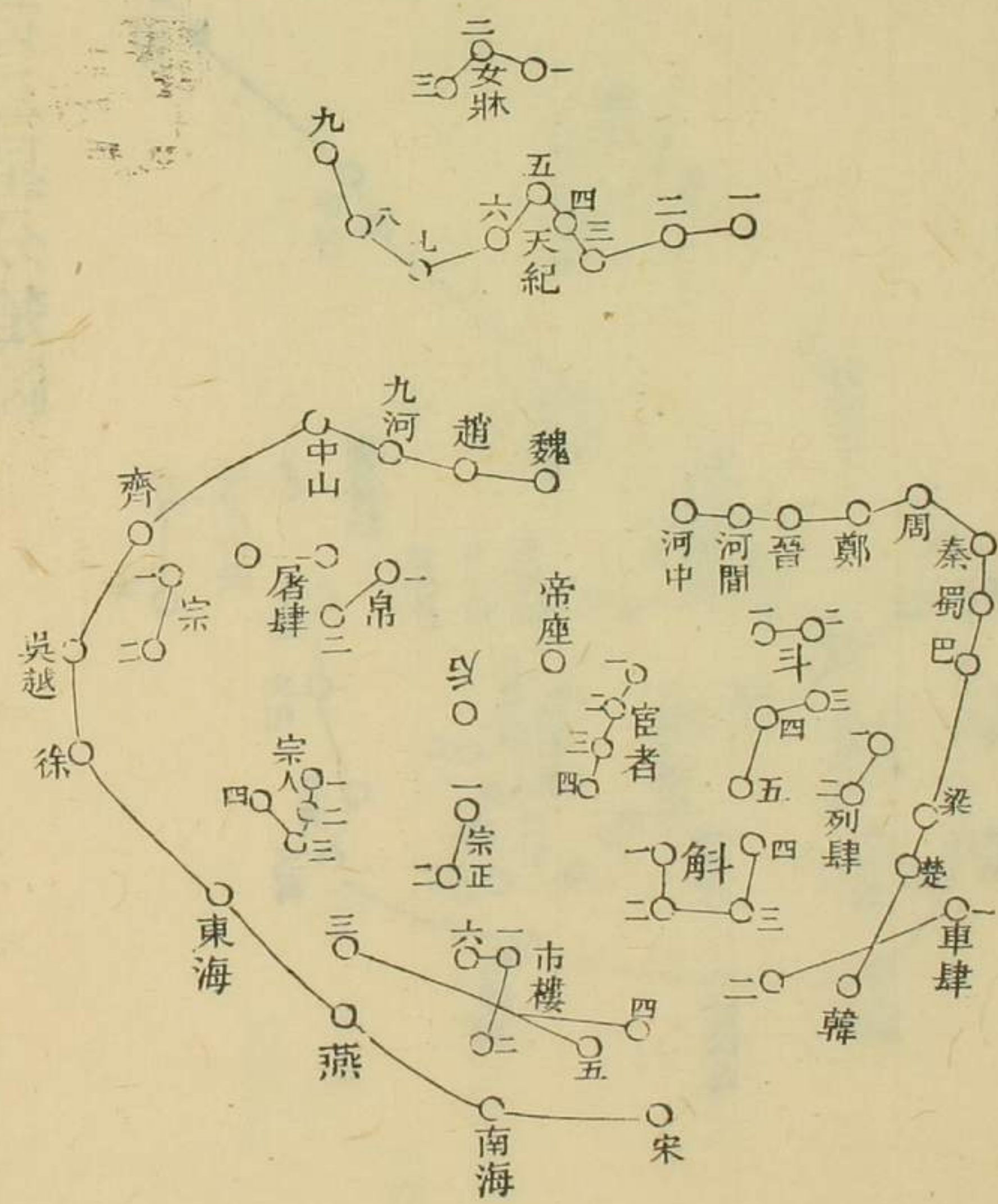
天市垣西蕃十一星分楚圖
