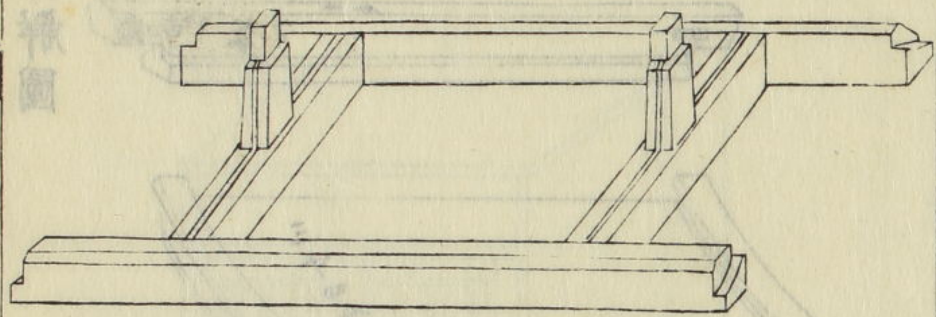
同架桁挿板圖
