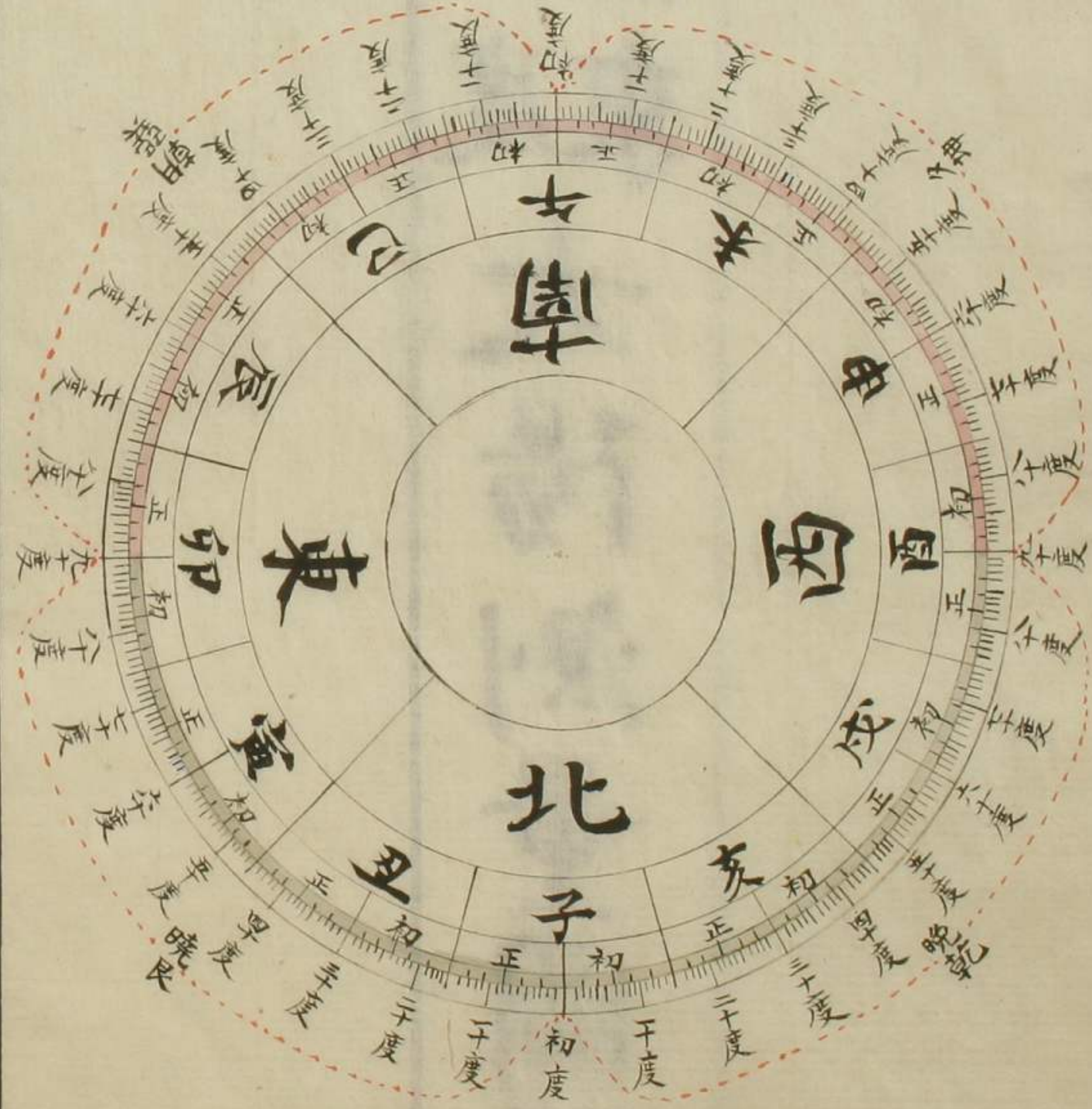
圖之度天合位方及分時
