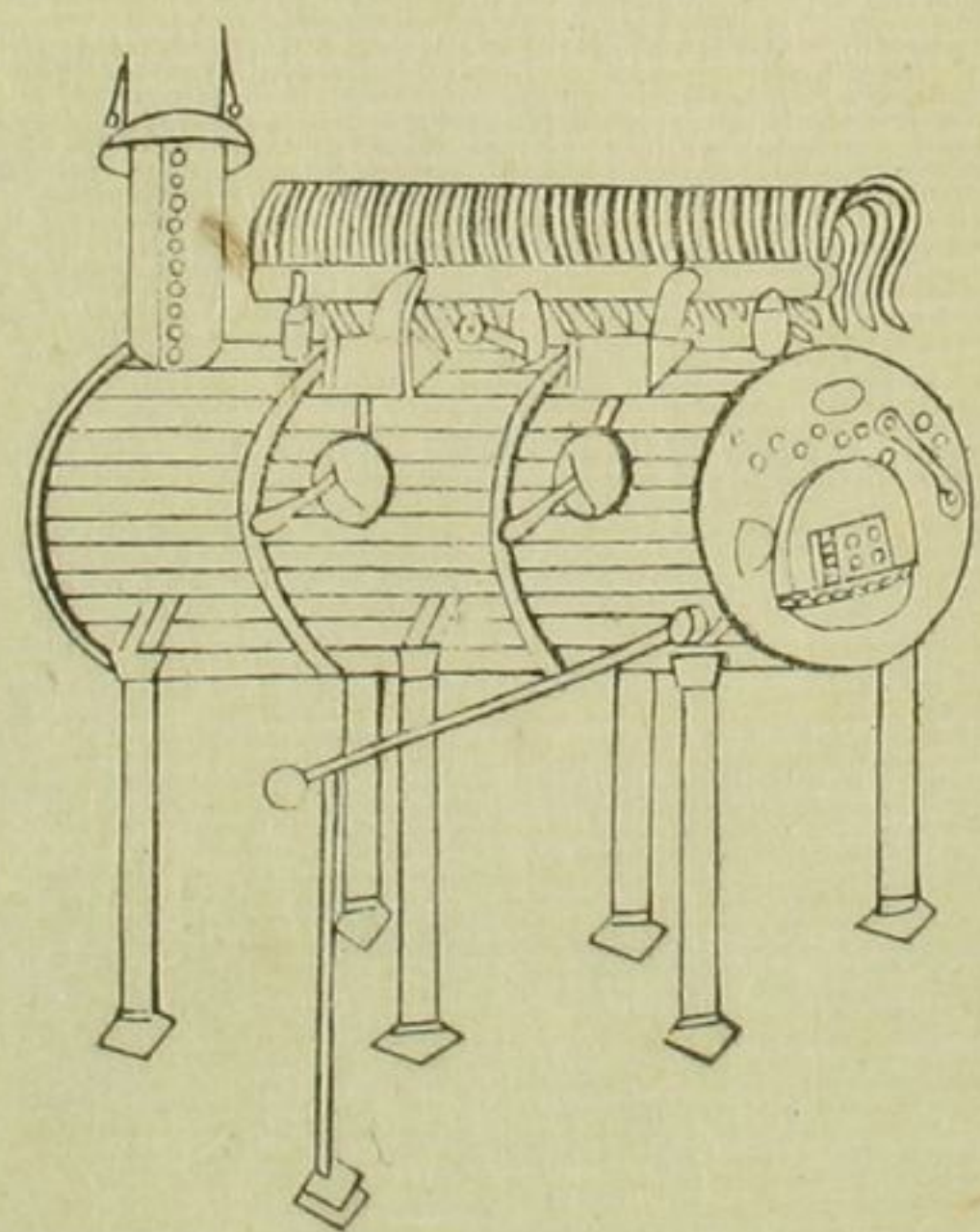
三十八 蒸汽 電機
