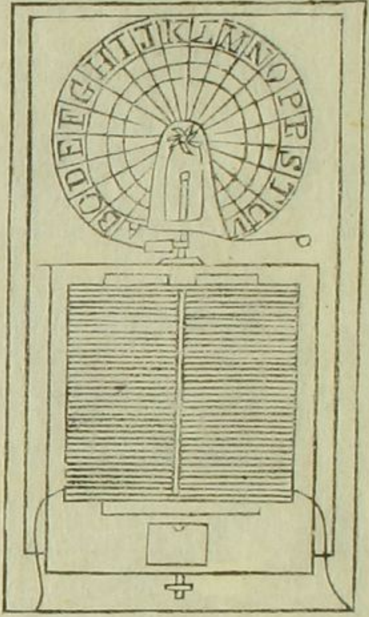
八十四 電報指 字機
