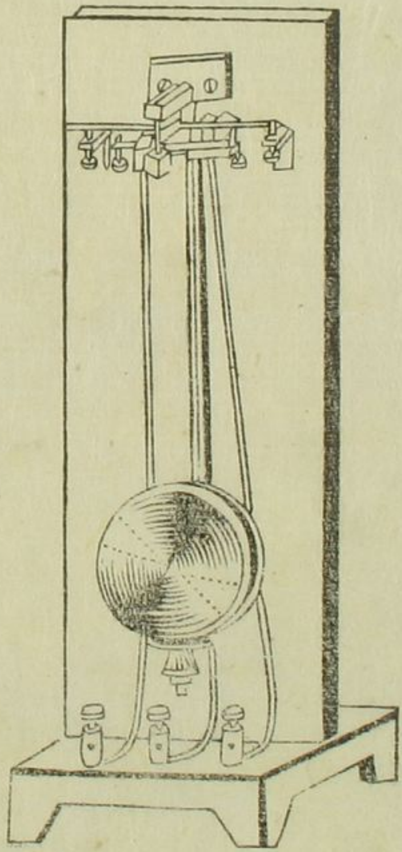
電鐘背 式 其面有 文紀時 有鐵指 字
