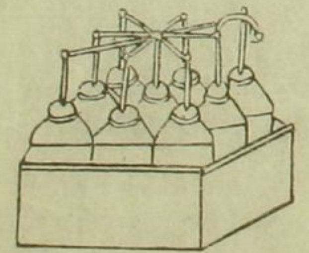
同上 數瓶相連
