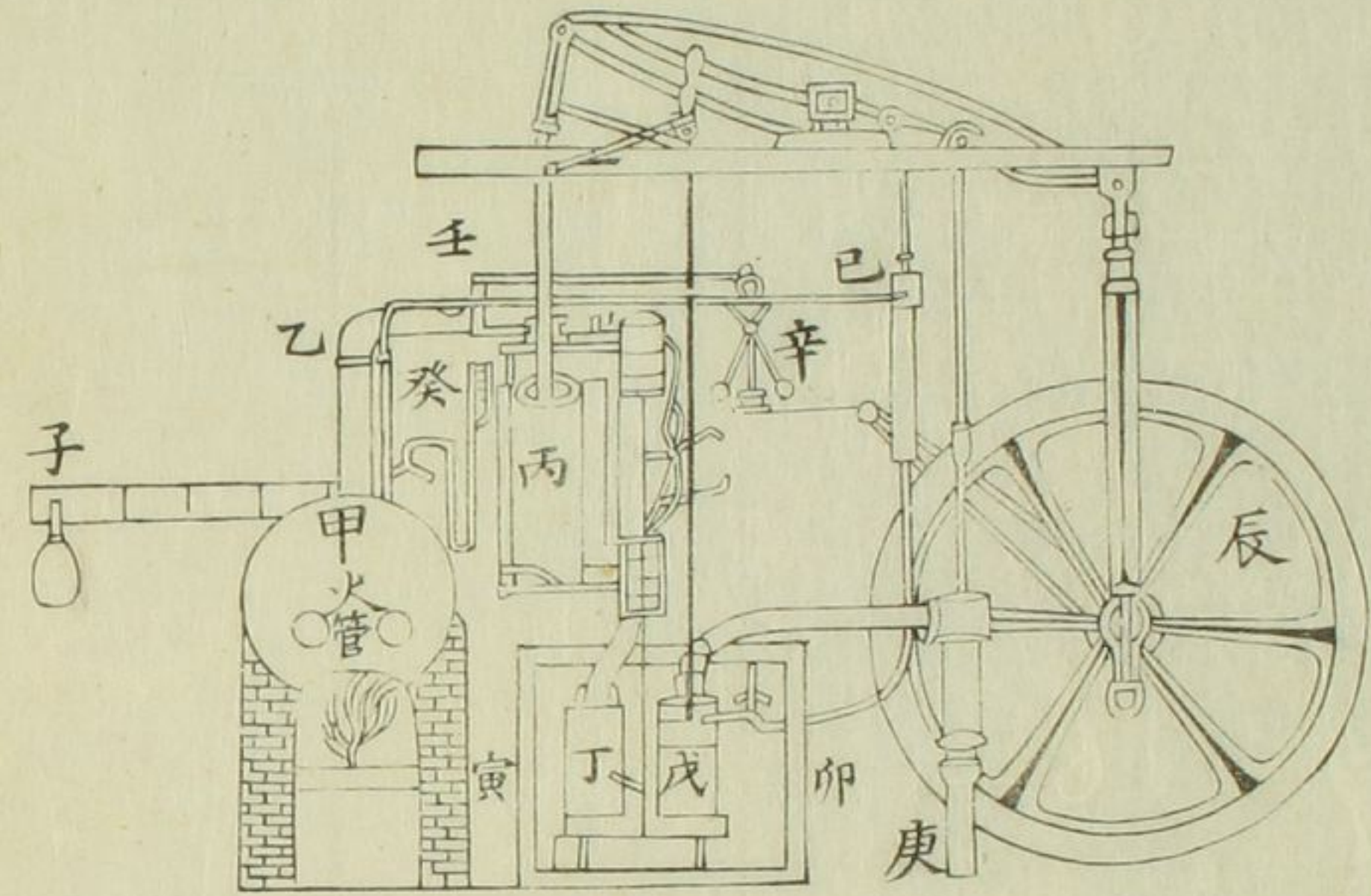
十五 氣機 全圖
