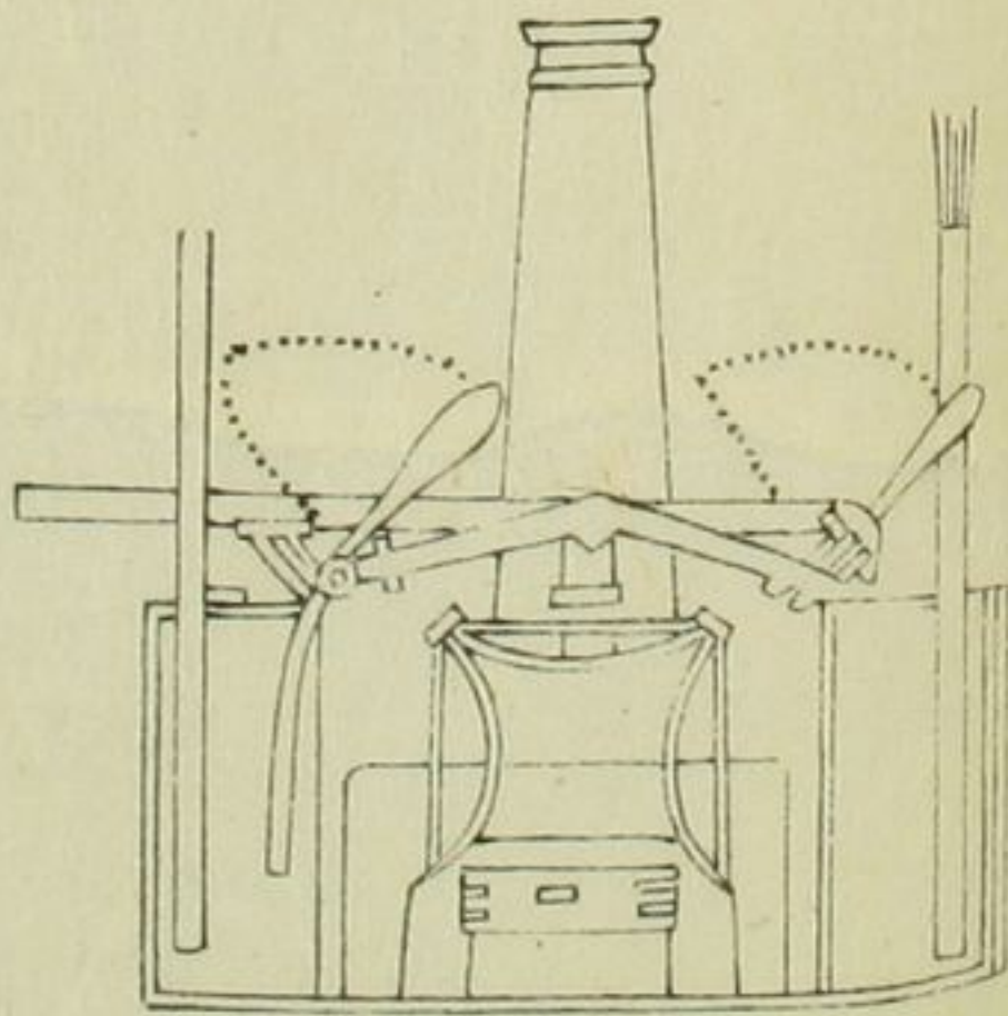
吳氏氣機 惟能催水
