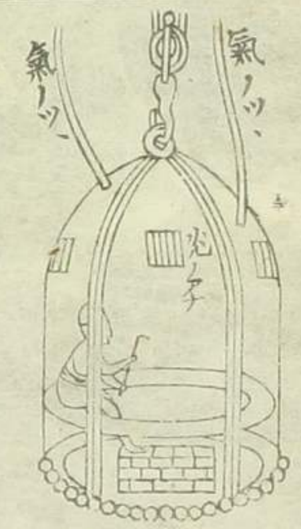
泳氣鐘ノ圖
