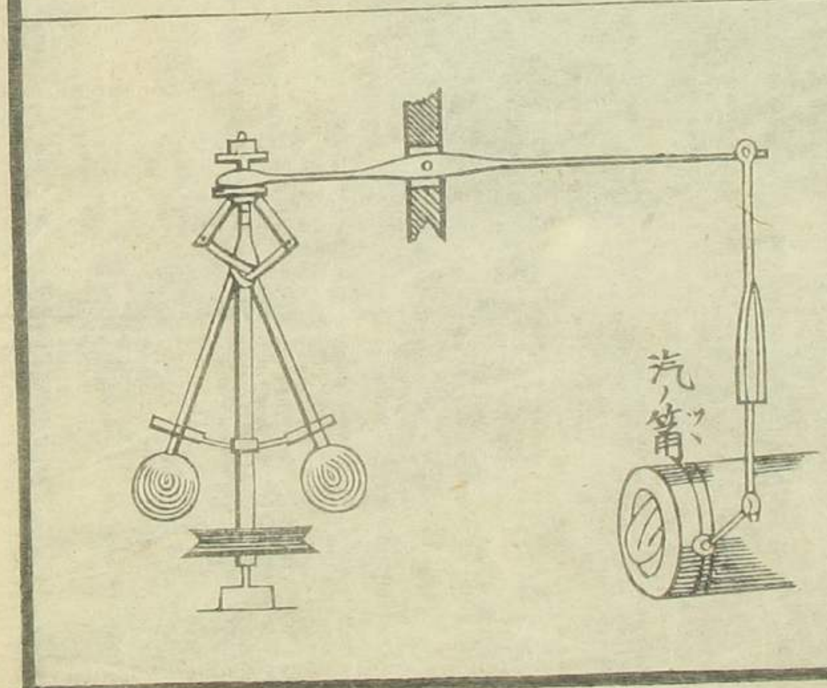
機ニテ圓キ球ヲ架タル圖
