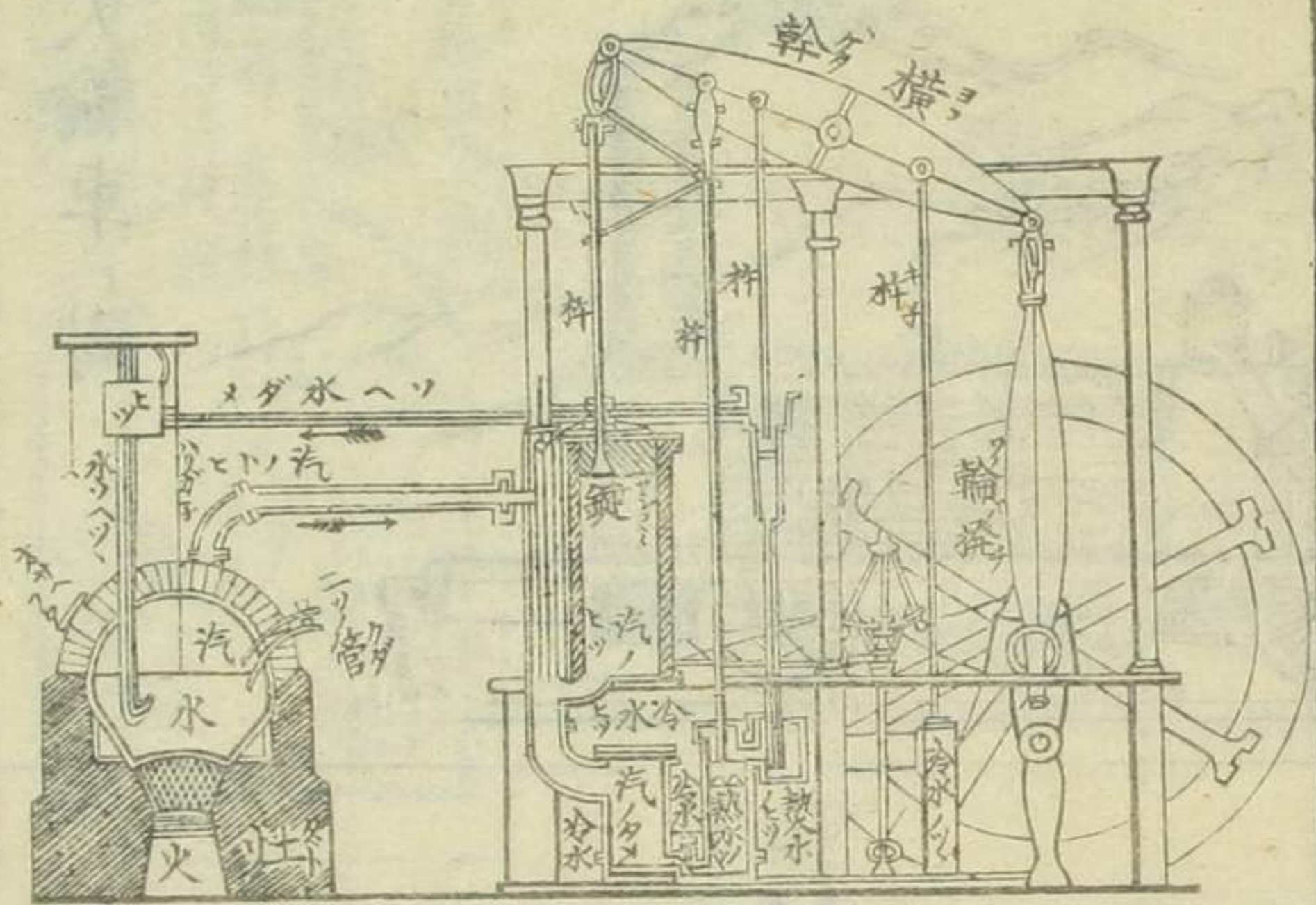
火輪機ノ圖
