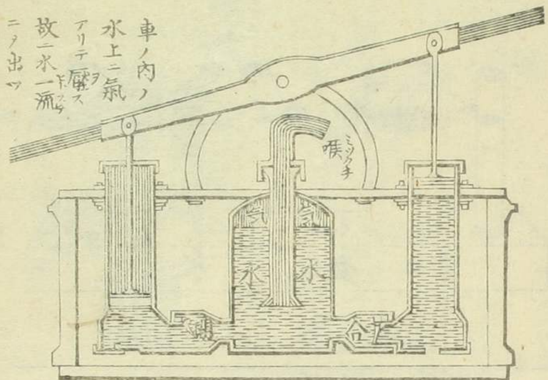
救火水車ノ圖
