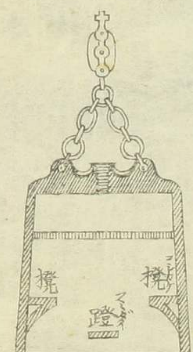
泳氣鐘ノ圖
