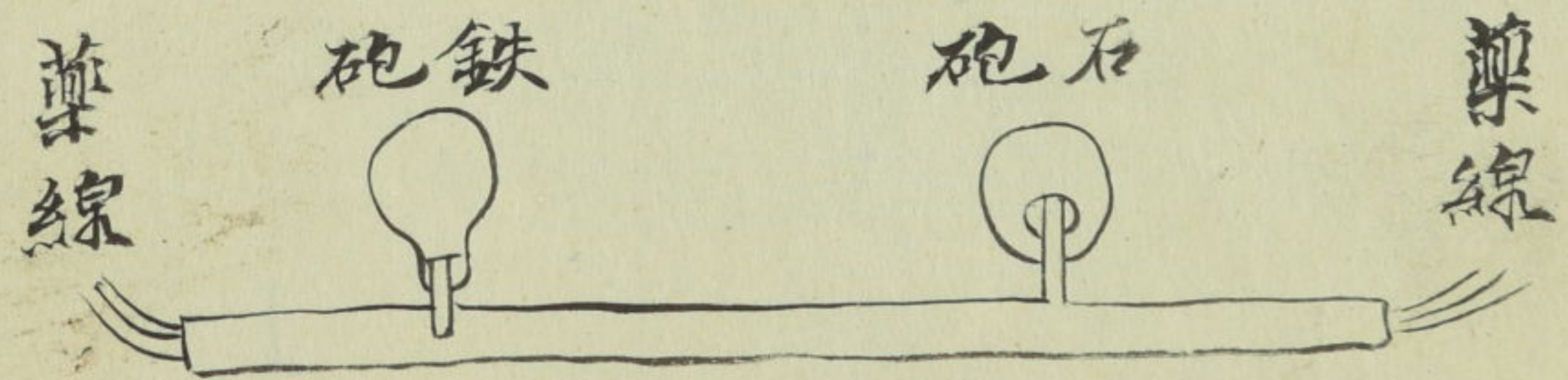
地坑埋伏石砲生鉄砲引藥線竹式
