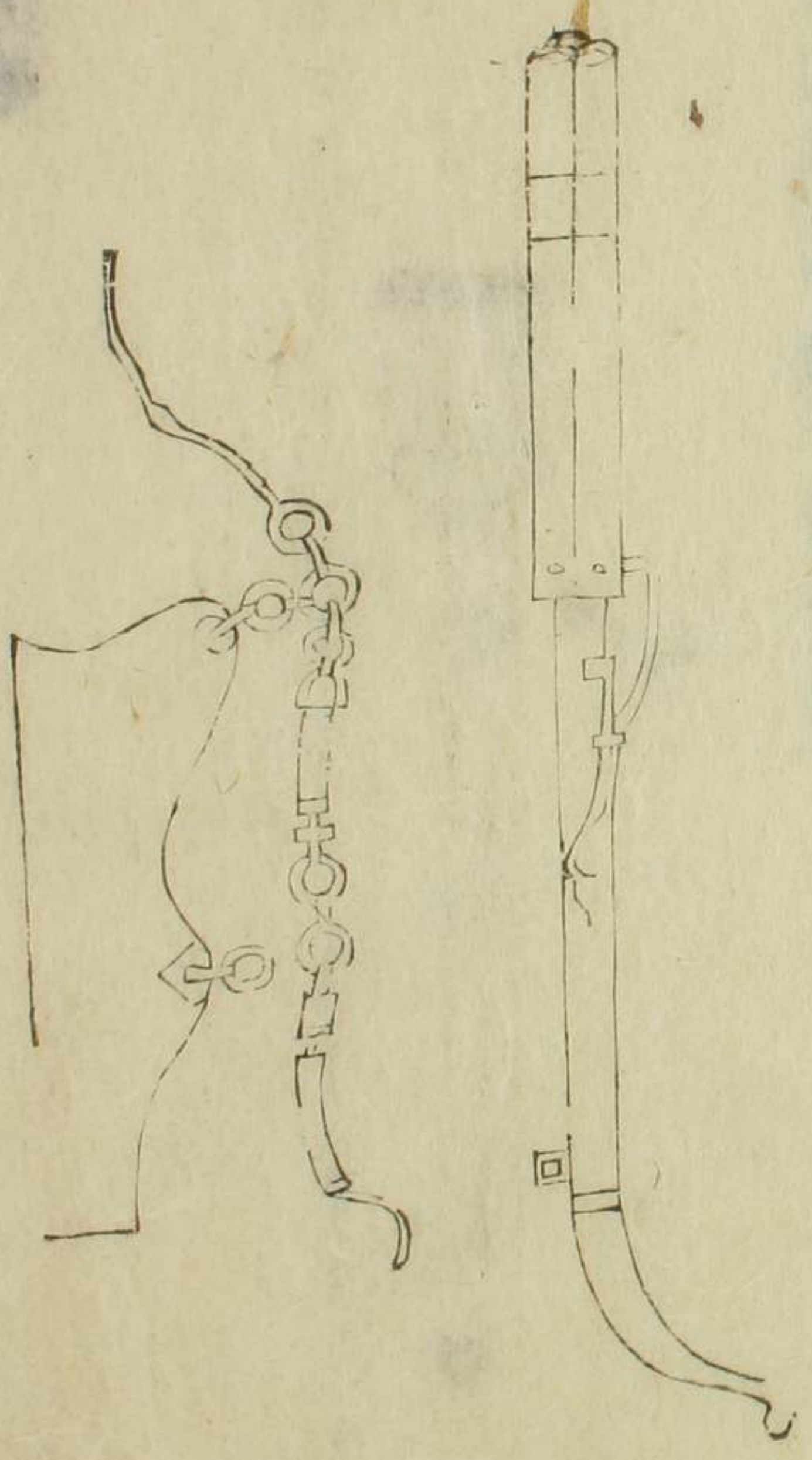
三捷神機 其製大約與五雷神機同
