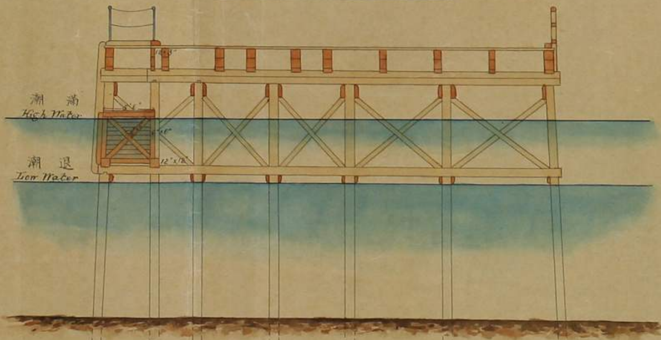
圖截橫之梯階
