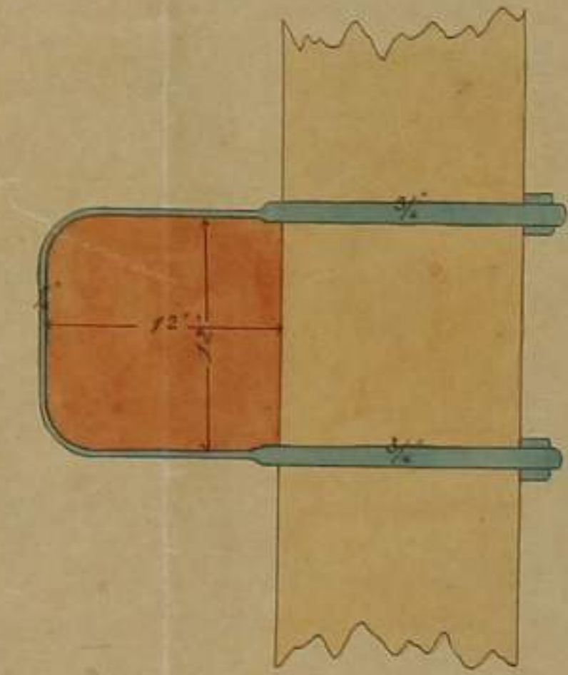
圖截橫部上木衝防
