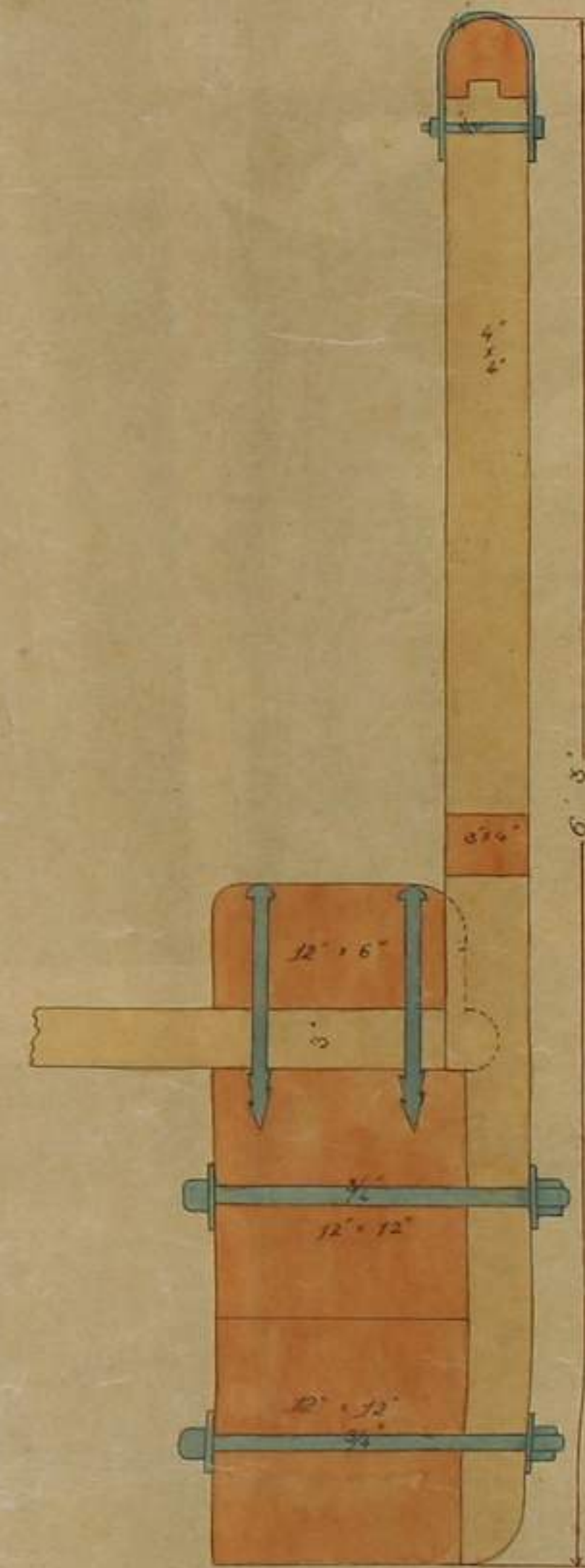
形立
