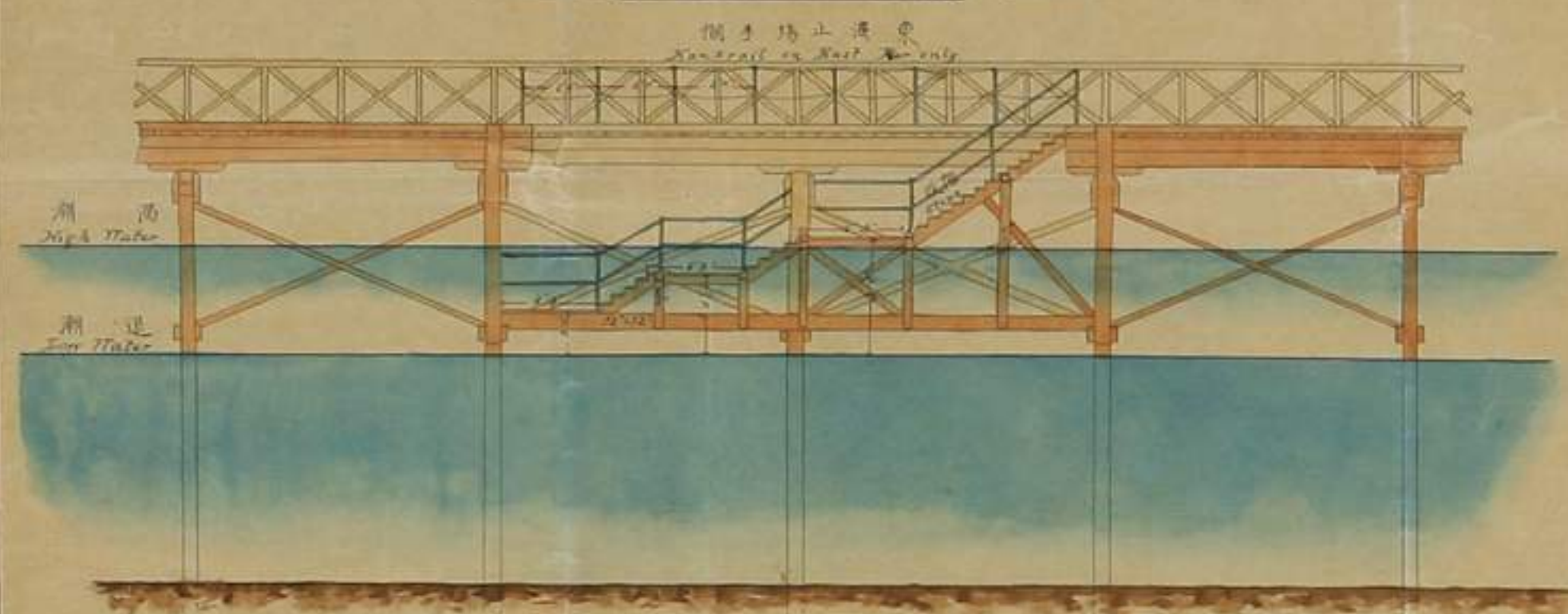
圖面平匡木梯階
