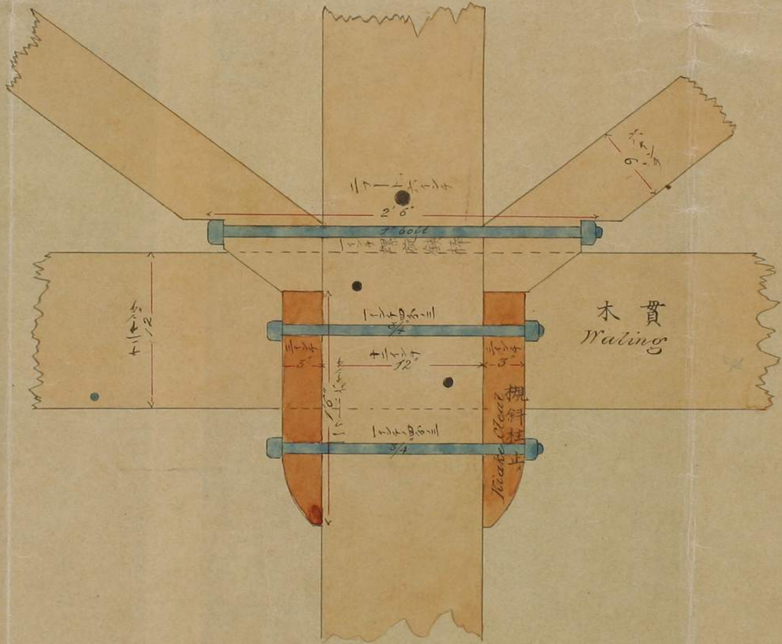
圖 截 橫 ——— CROSS SECTION ———
