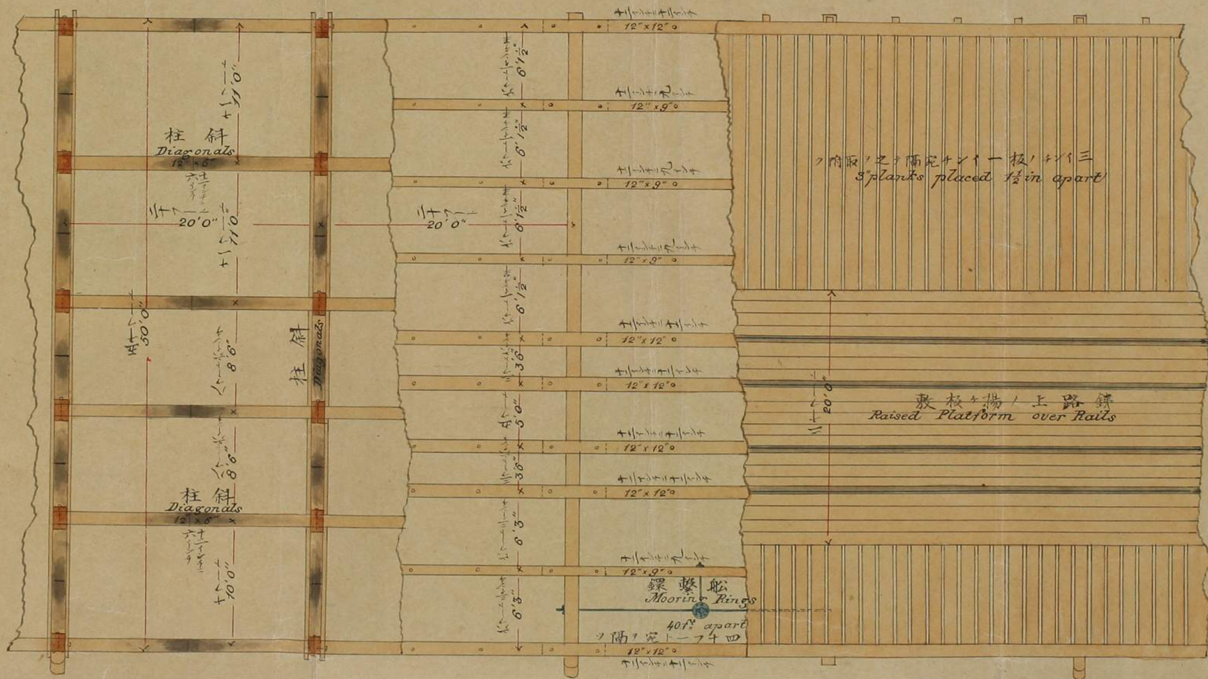
圖面平 PLAN
