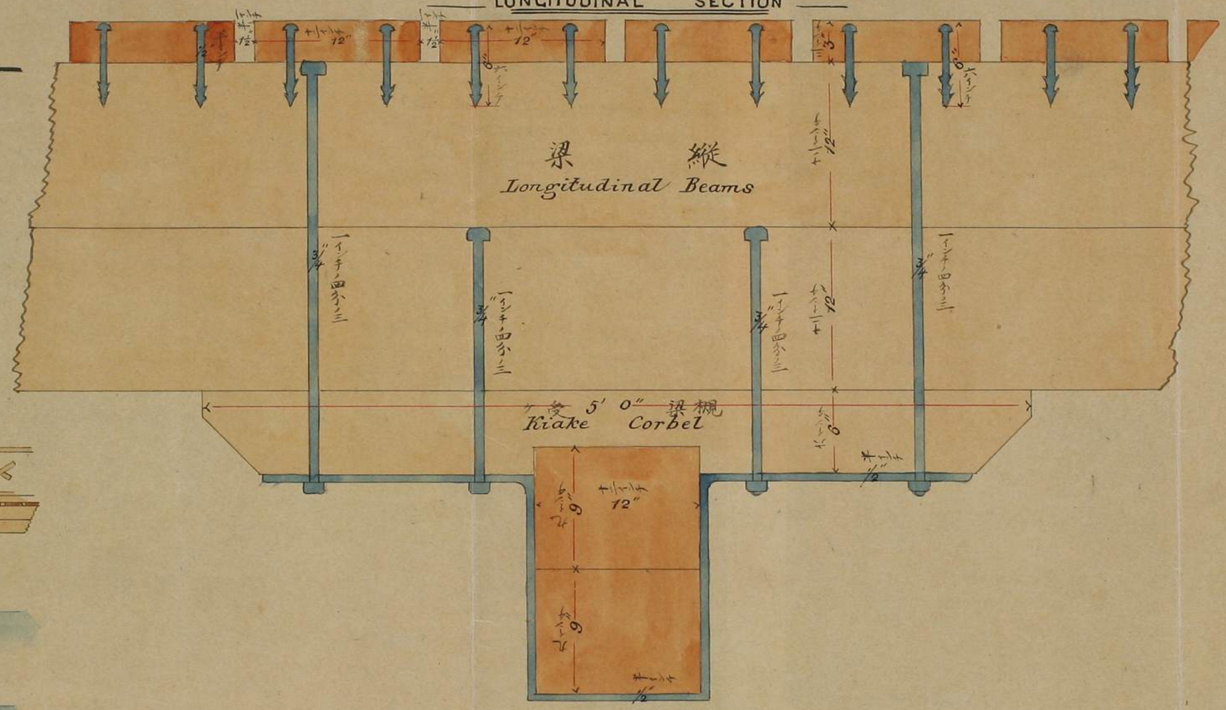
組 梁 CROSSING OF BEAMS
