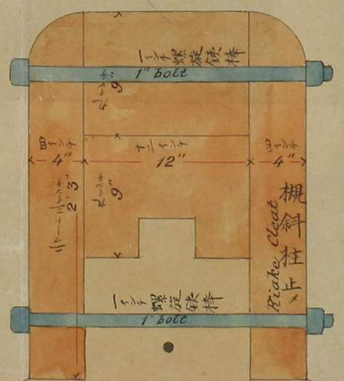
圖 截 縱 LONGITUDINAL SECTION
