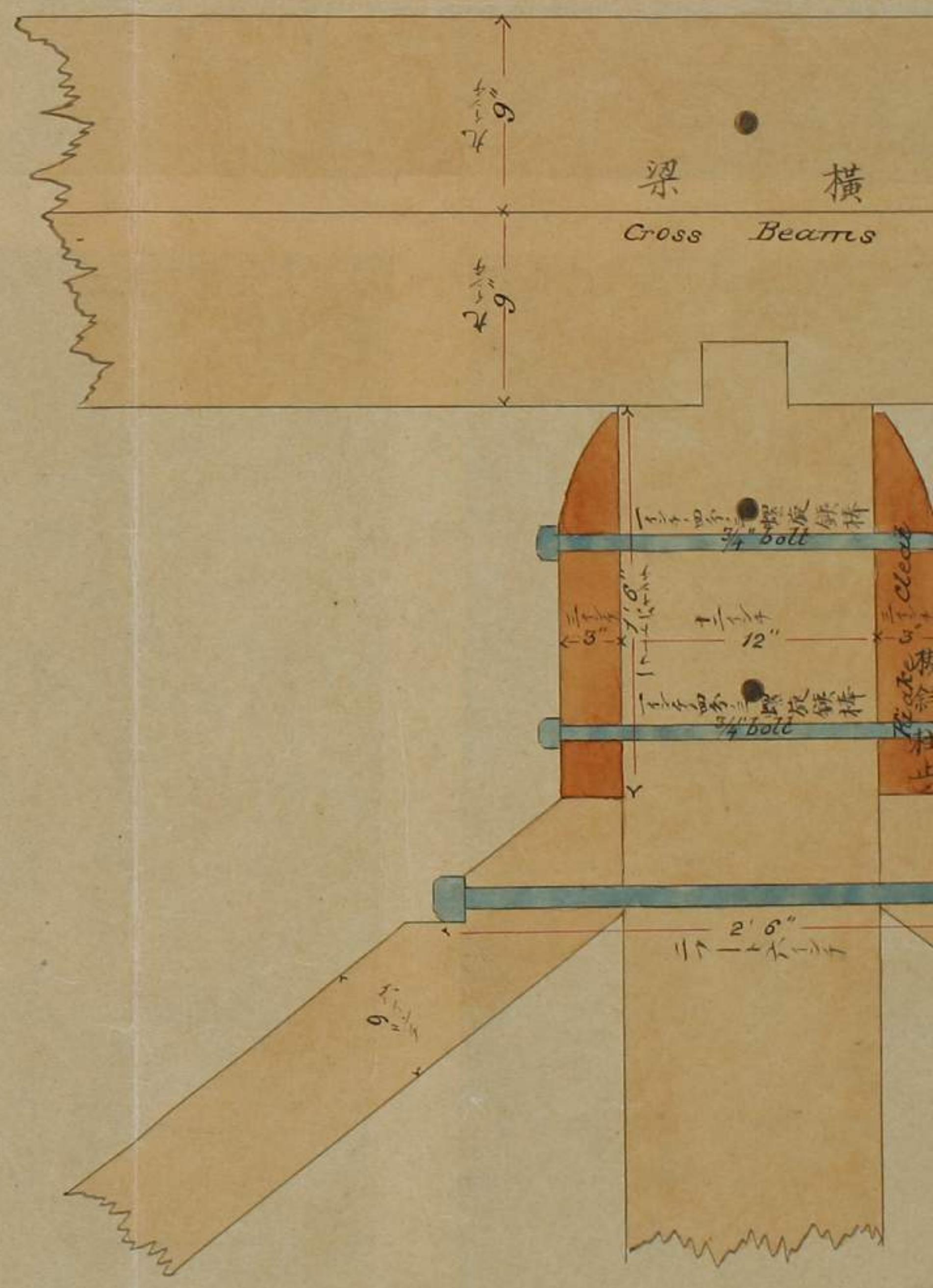
底 架 木 BOTTOM OF FRAMEWORK
