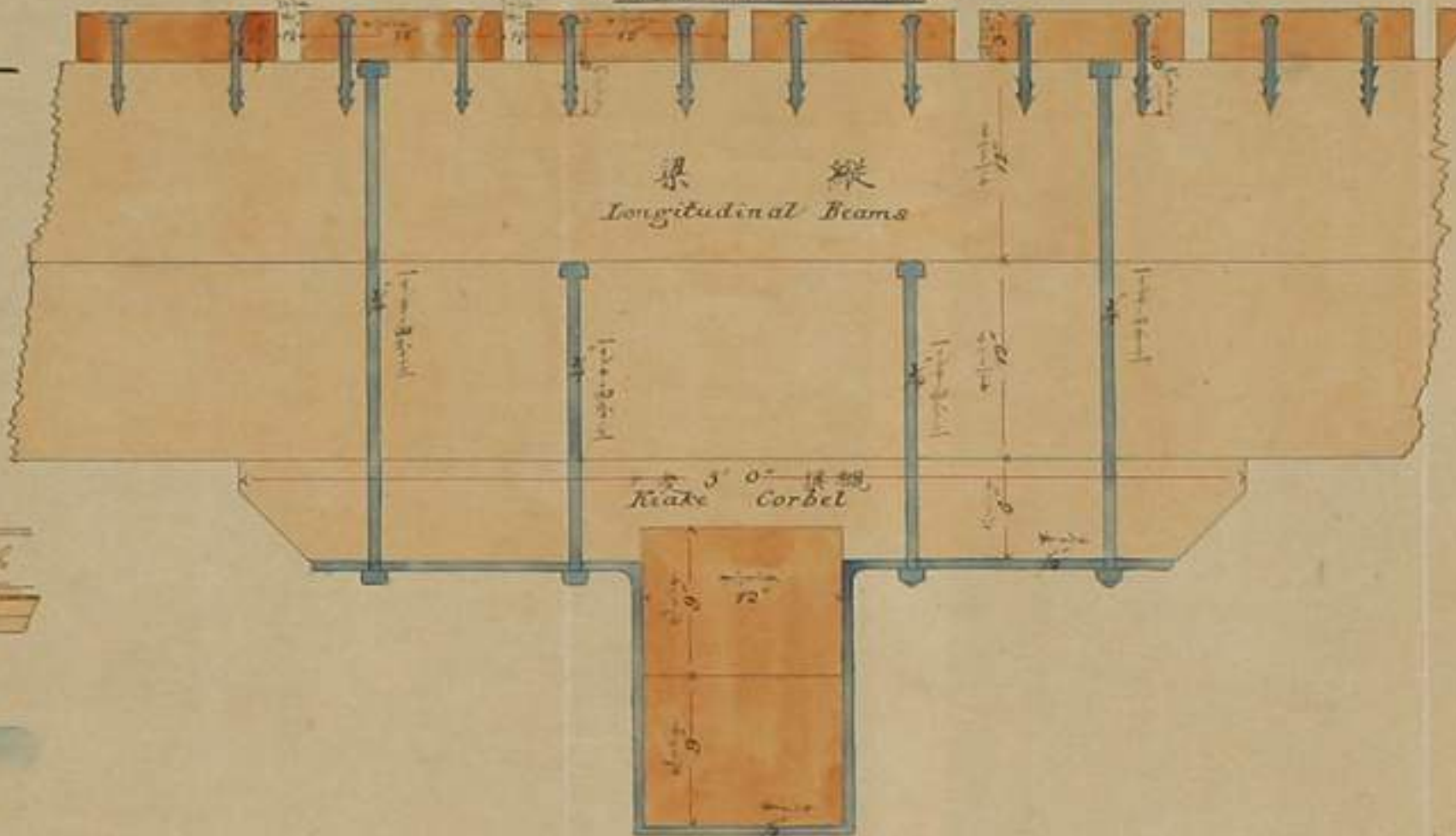
圖截縱 LONGITUDINAL SECTION
