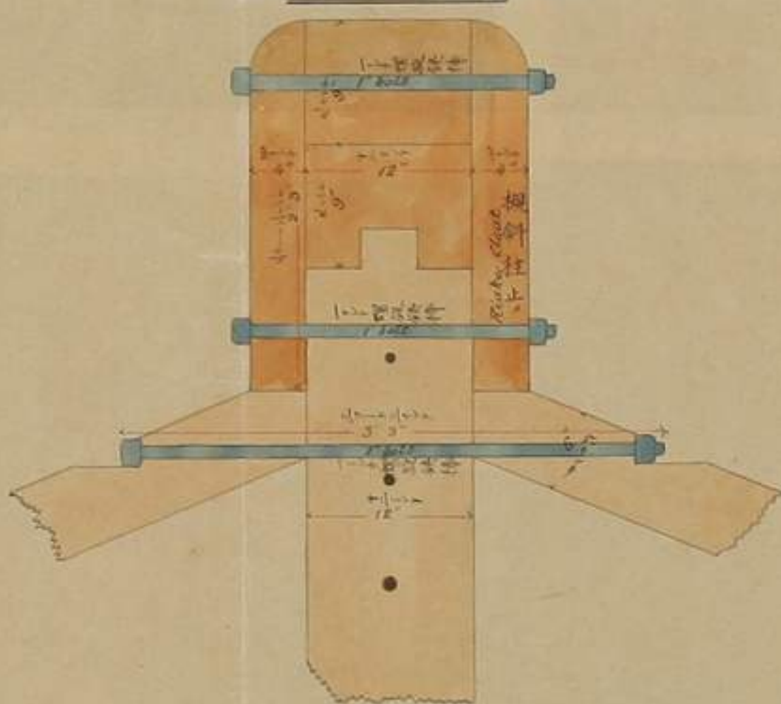
圖截縱 LONGITUDINAL SECTION
