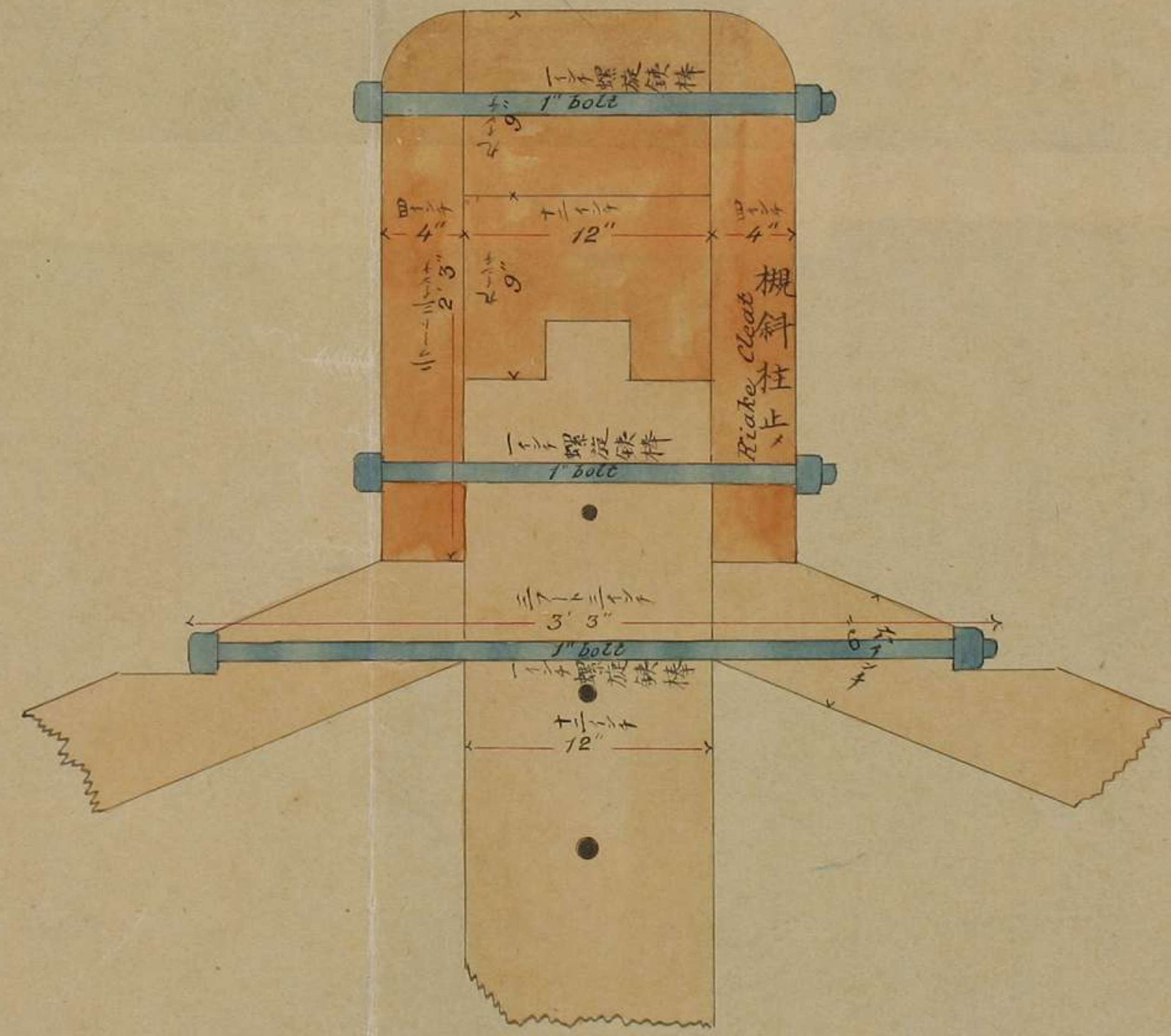
圖 截 縱 LONGITUDINAL SECTION
