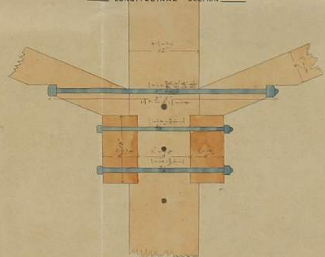
圖截縱 LONGITUDINAL SECTION
