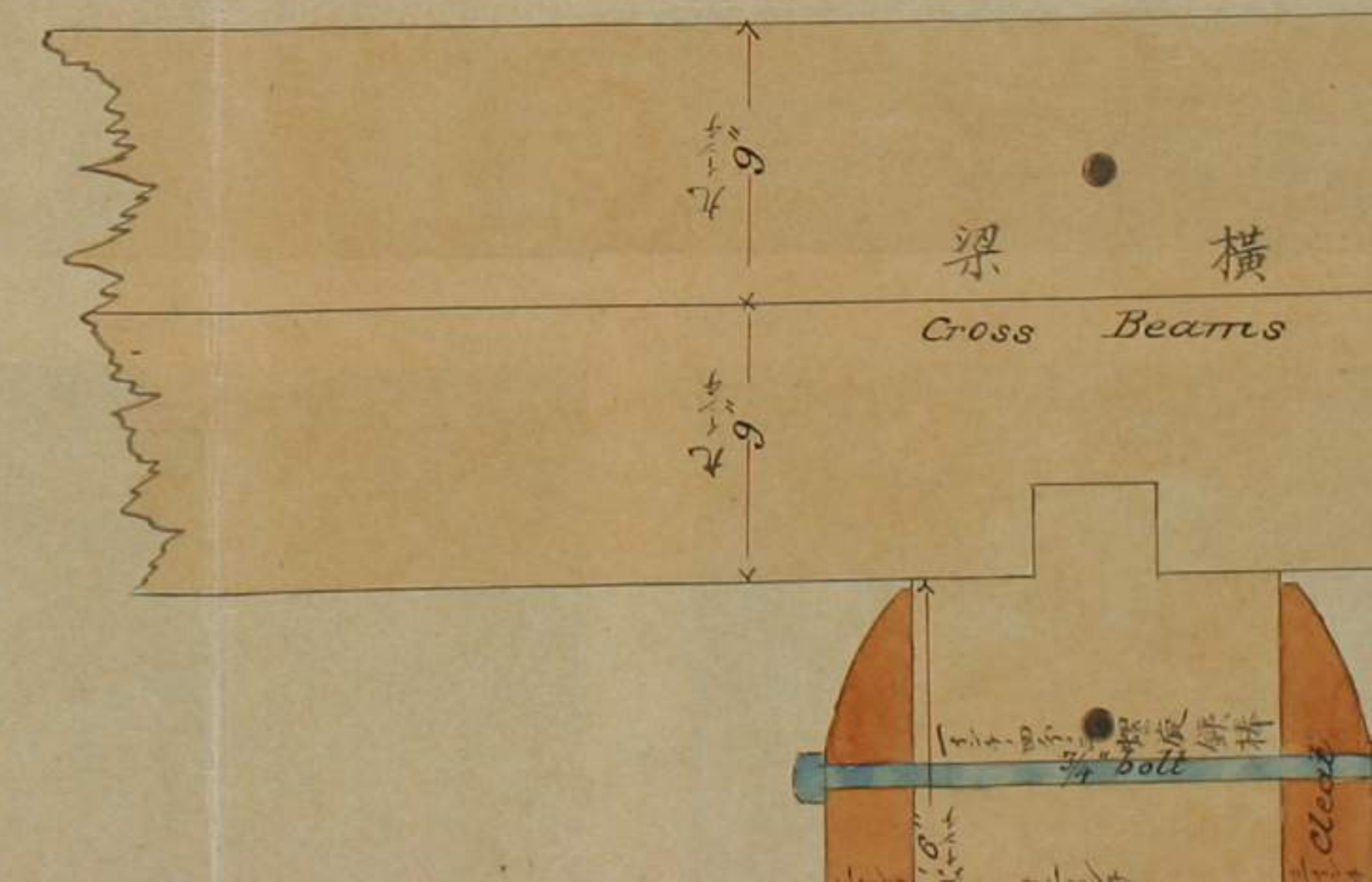
圖 截 橫 CROSS SECTION
