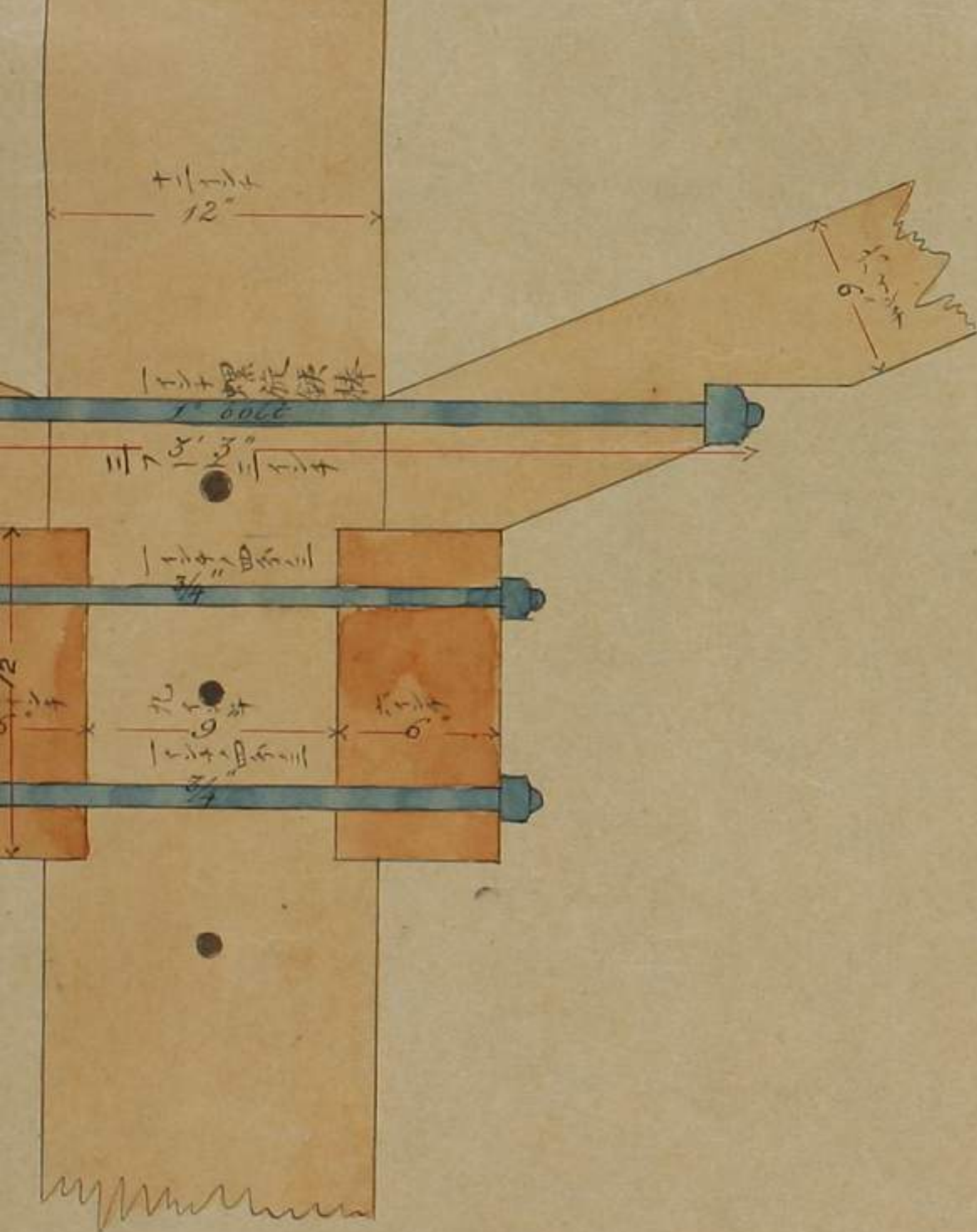
圖 截 縱 ——— LONGITUDINAL SECTION ———
