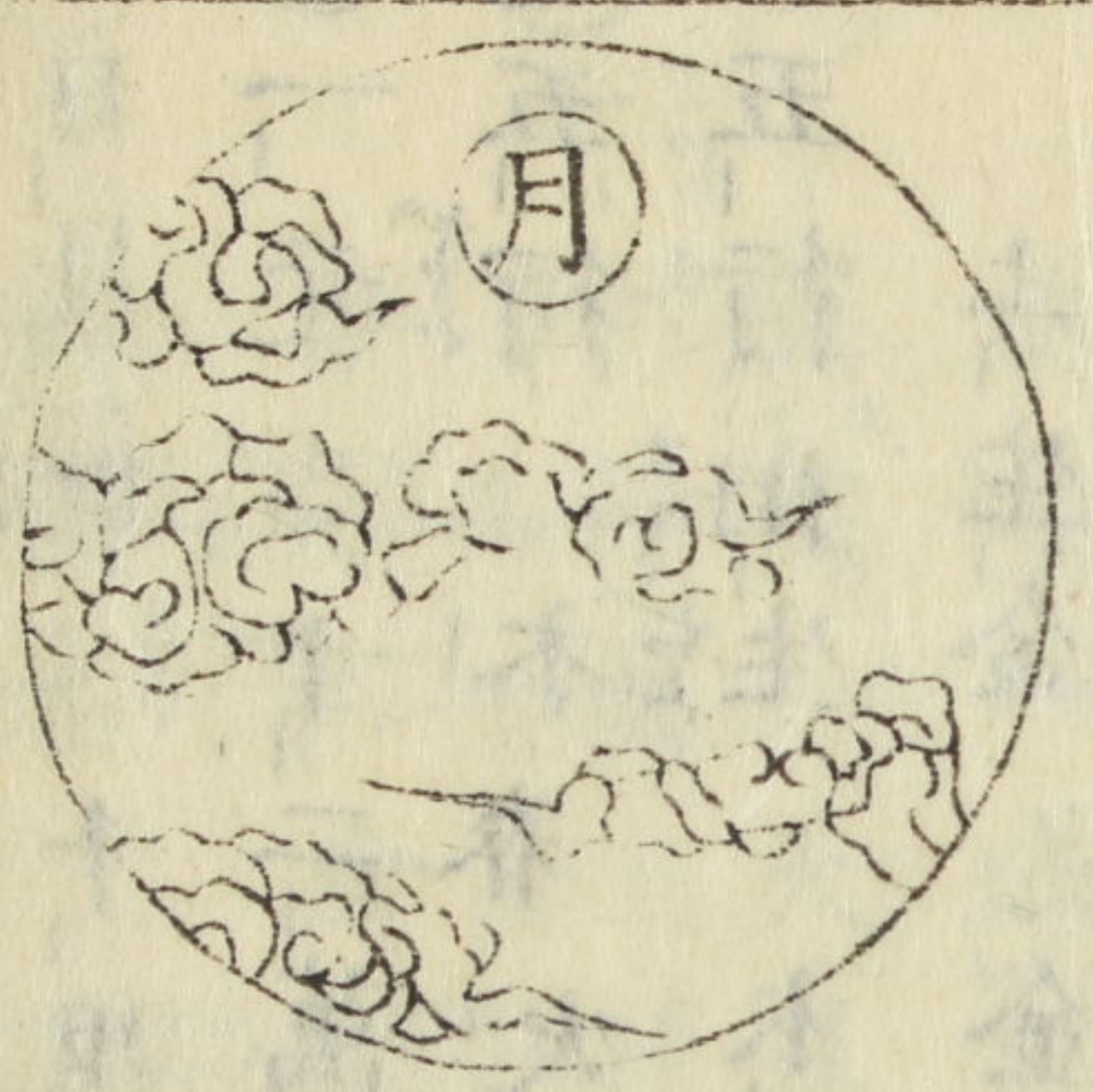
月蝕之圖
