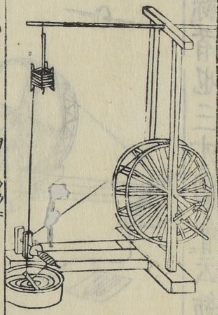
紡車
