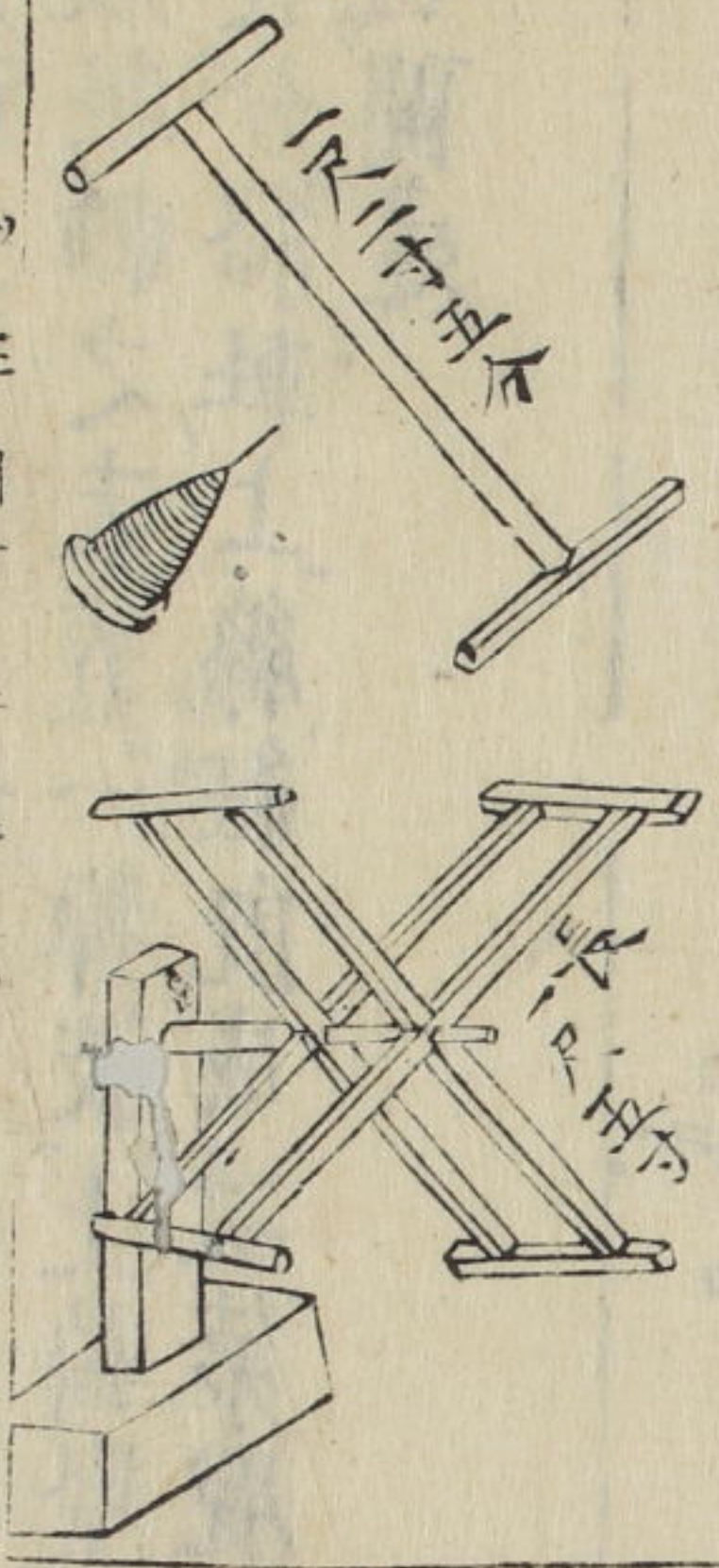
蟠車
