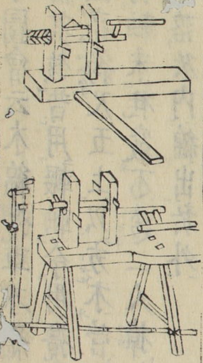
攪車
