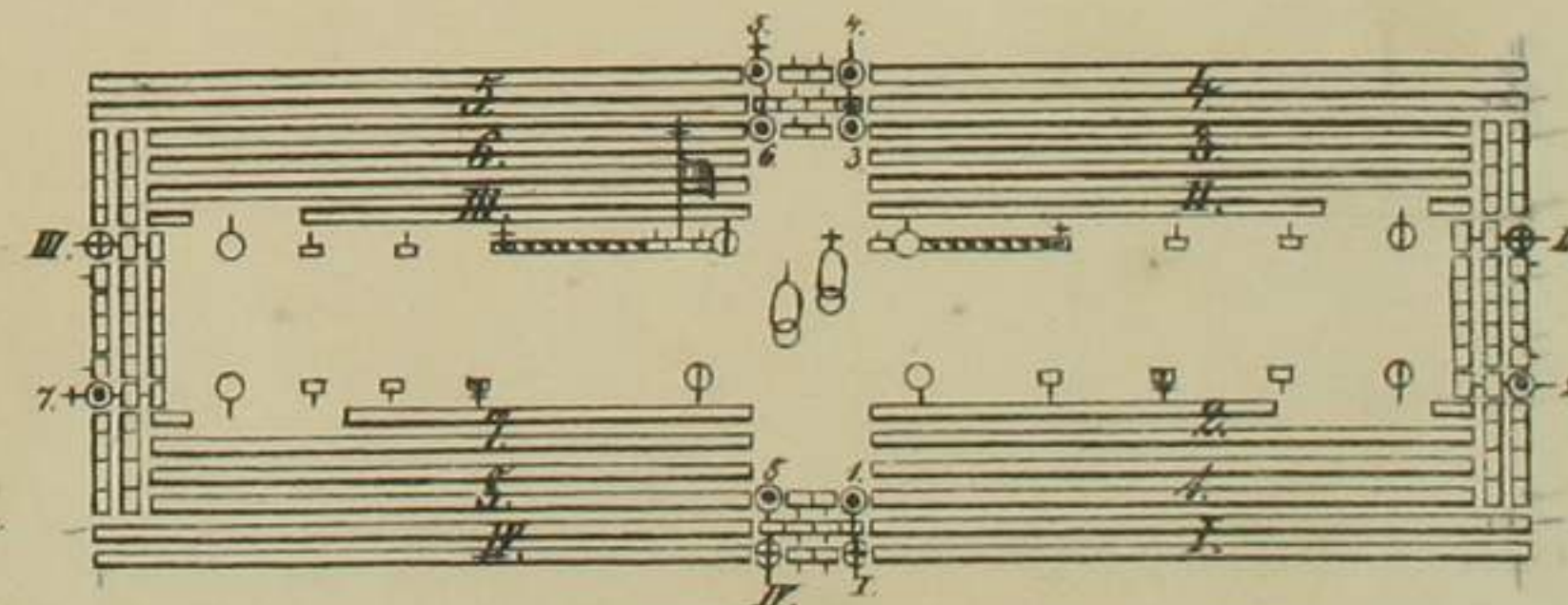
Fig. 16. Das Bataillons-Carree.
