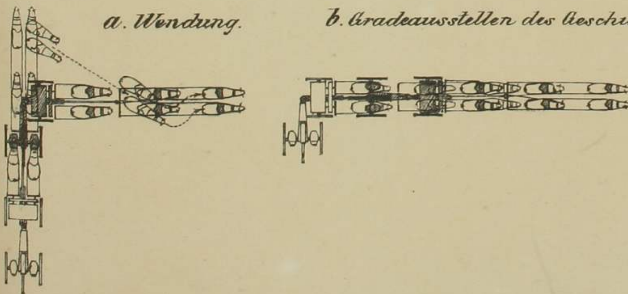
Fig. 19. Hakenwendung Rechtsum.
