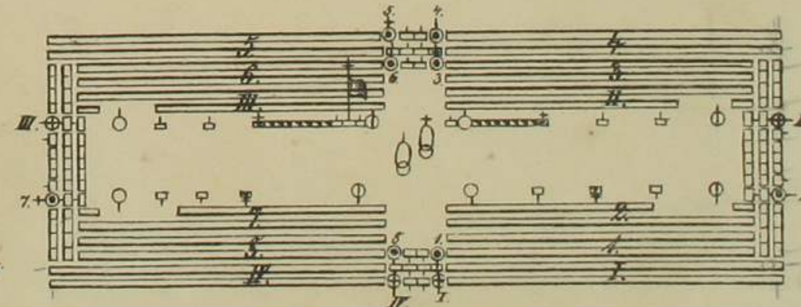
Fig. 16. Das Bataillons-Carree.
