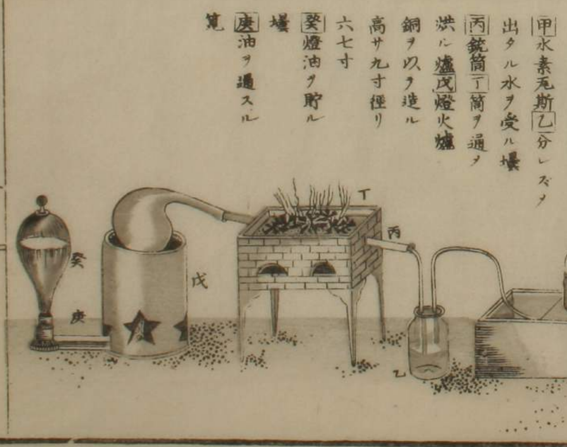
第二圖 分離水式
