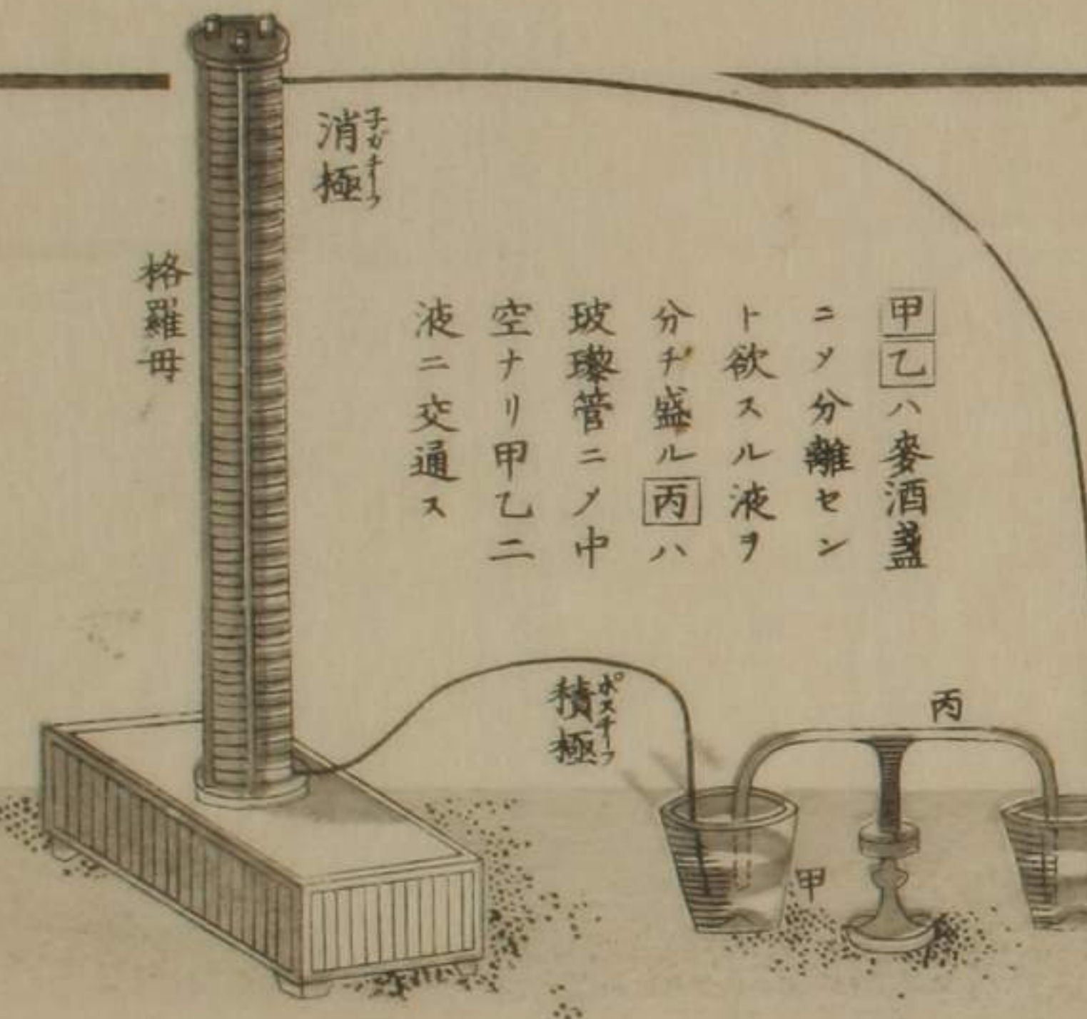
第七圖 以福爾答攝格羅母分離亞爾加里式
