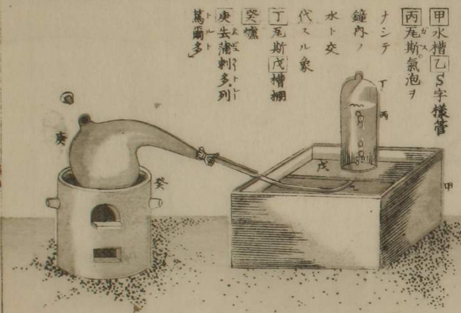
第一圖 聚氣裝置
