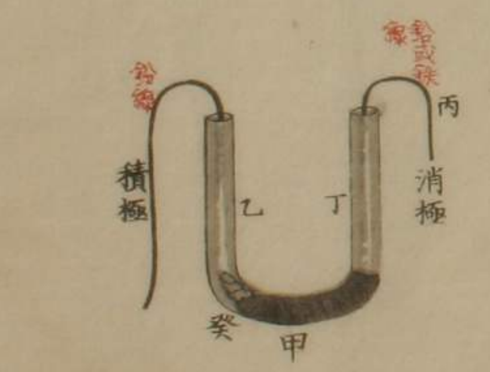
第九圖 務爾斯的度氏瓦爾華尼機
