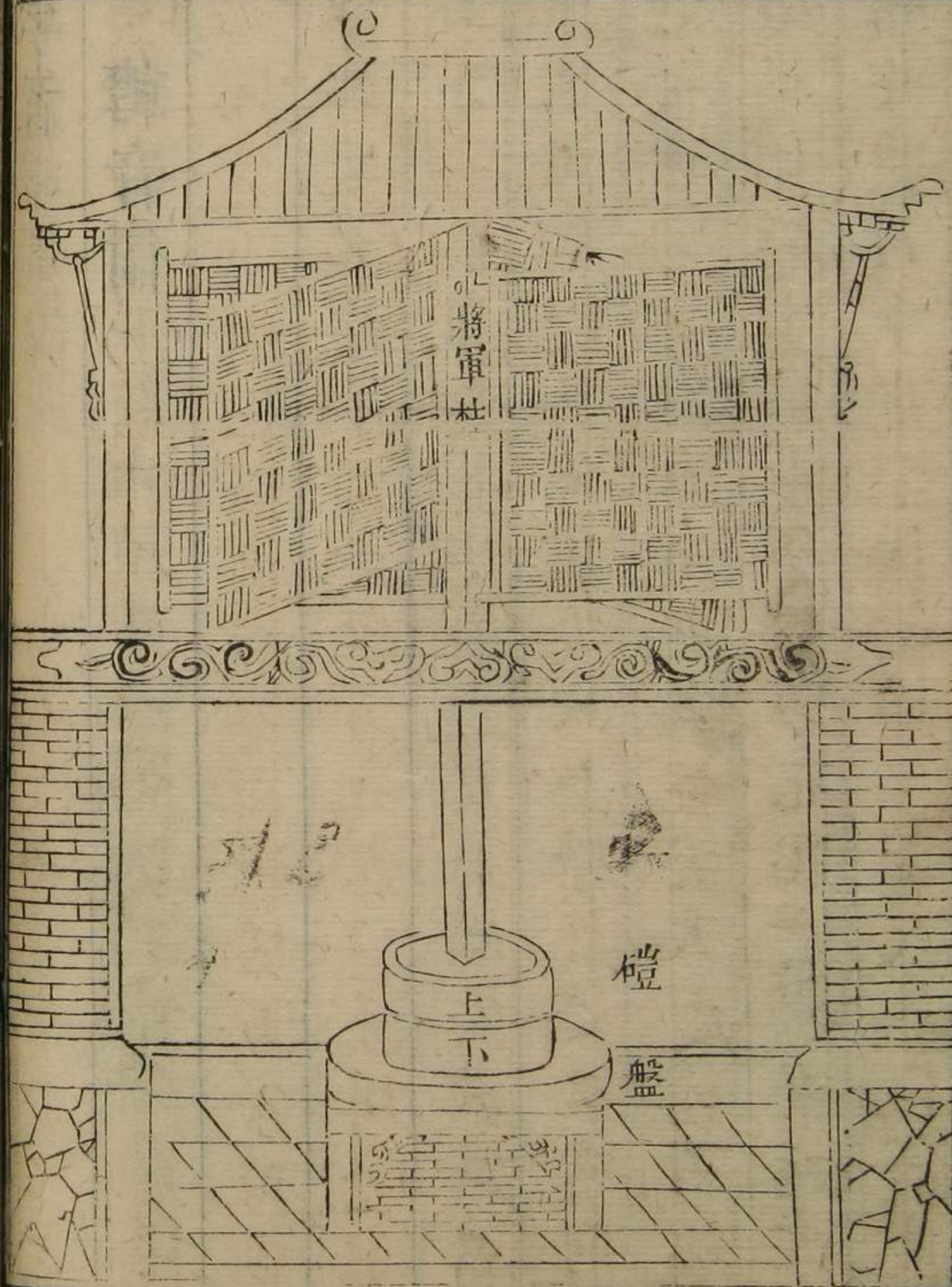
風磴圖說
