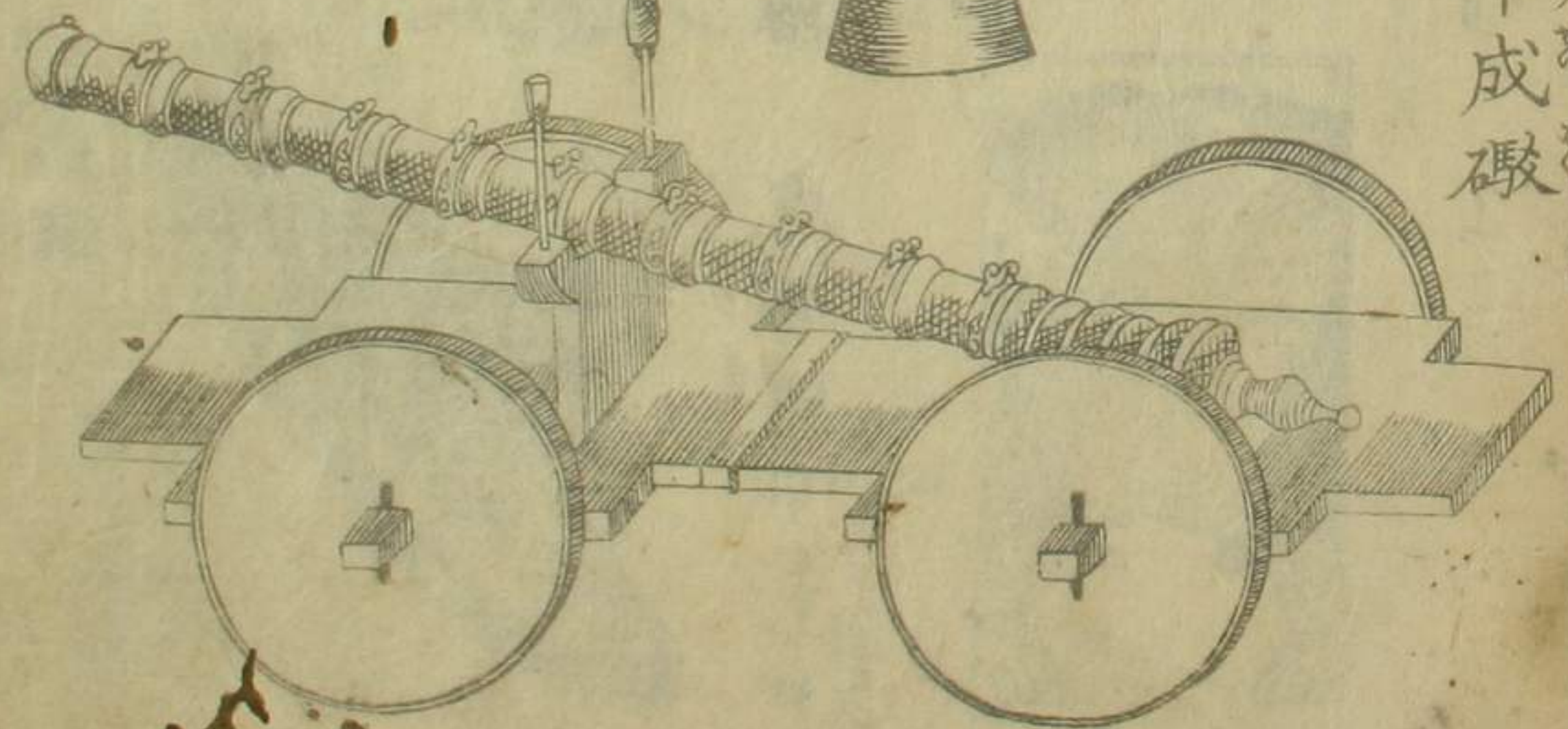
行營信礮
